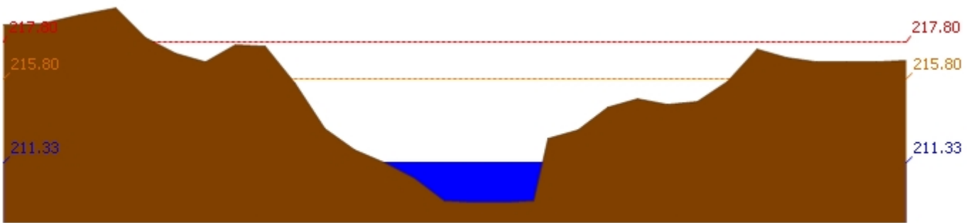
สถานี 120205T แม่น้ำป่าสักที่บ้านอู่กะทาด ต.ศิลา อ.หล่มเก่า จ.เพชรบูรณ์ ระดับน้ำ 211.33 ม.รทก.
