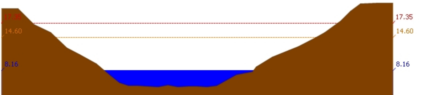
สถานี 120109T แม่น้ำป่าสักที่ อ.แก่งคอย ต.แก่งคอย อ.แก่งคอย จ.สระบุรี ระดับน้ำ 8.16 ม.รทก.
