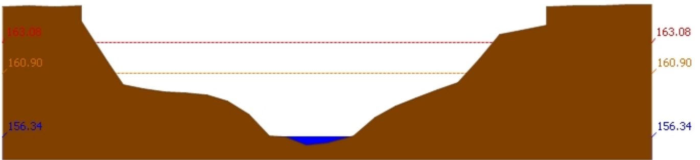
สถานี 120105T แม่น้ำป่าสักที่บ้านวังมเสหนือ ต.ทำอัญญ อ.หล่มสัก จ.เพชรบูรณ์ ระดับน้ำ 156.34 ม.รทก.
