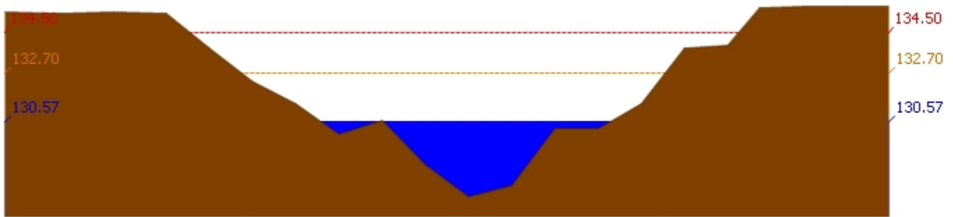
สถานี 120111T แม่น้ำป่าสักที่บ้านจางวาง ต.ลานบัว อ.หล่มสัก จ.เพชรบูรณ์ ระดับน้ำ 130.57 ม.รทก.
