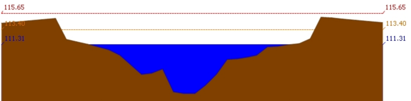
สถานี 120107T แม่น้ำป่าสักที่ อ.เมืองเพชรบูรณ์ ต.นาป่า อ.เมือง จ.เพชรบูรณ์ ระดับน้ำ 111.31 ม.รทก.
