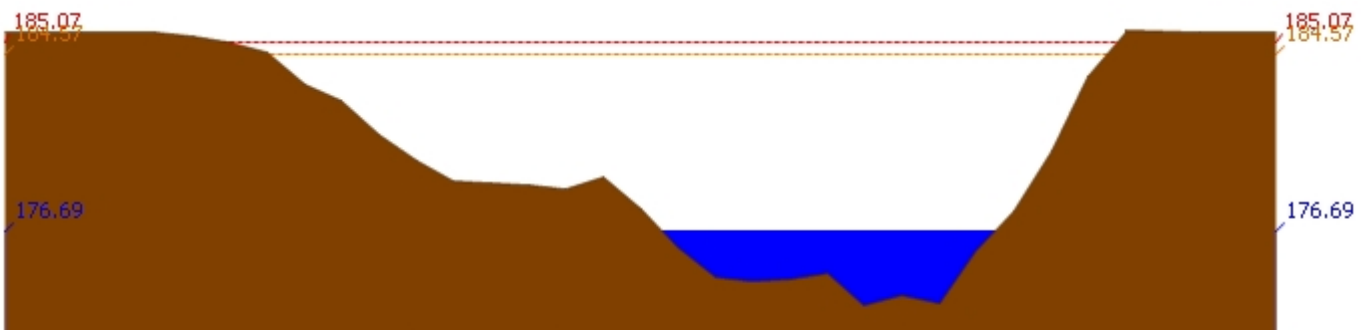
สถานี 070116T แม่น้ำวังที่บ้านแม่เตี๊ยะ ต.แม่ถอด อ.เถิน จ.ลำปาง ระดับน้ำ 176.69 ม.รทก.
