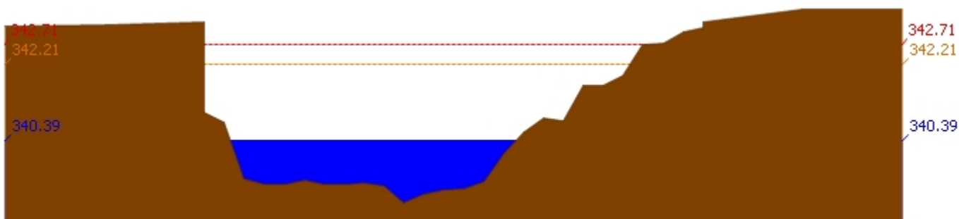
สถานี 070304T น้ำแม่สอยที่บ้านหนองกอก ต.แม่สุก อ.แจ้ห่ม จ.ลำปาง ระดับน้ำ 340.39 ม.รทก.
