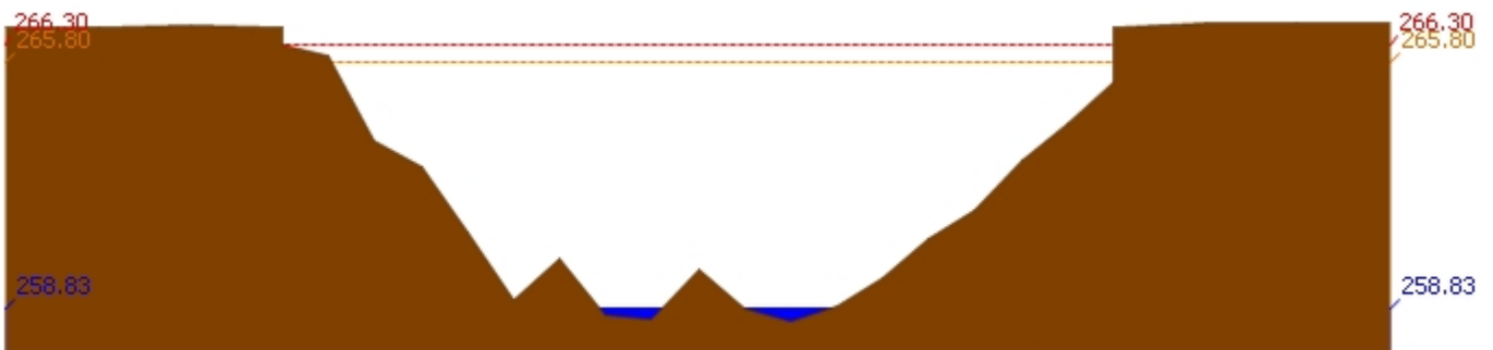
สถานี 070604T น้ำแม่จางที่บ้านสุใหม่โขมยมงคล ต.หัวเสือ อ.แม่ทะ จ.ลำปาง ระดับน้ำ 258.83 ม.รทก.
