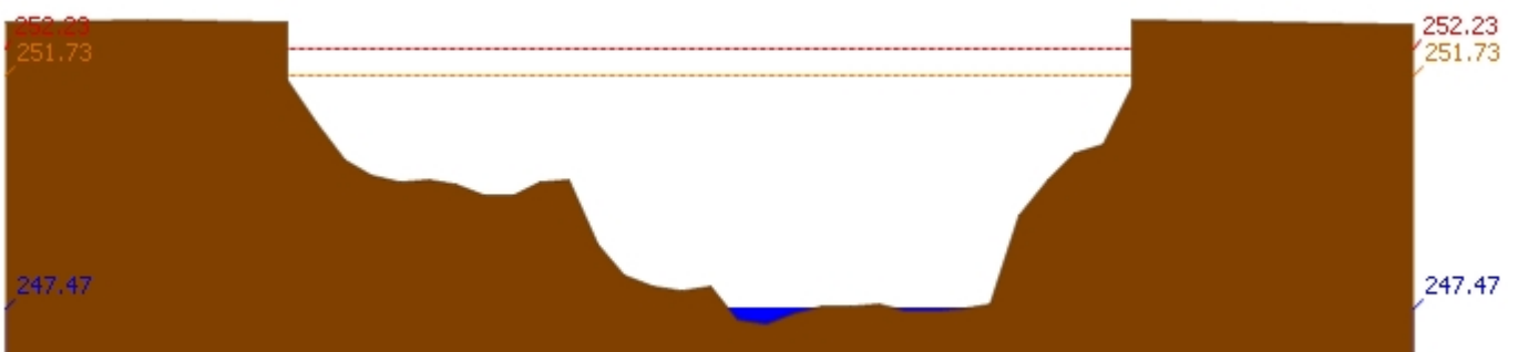
สถานี 070403T น้ำแม่ตุ๋ยที่บ้านแค ต.บ้านเป้า อ.เมืองลำปาง จ.ลำปาง ระดับน้ำ 247.47 ม.รทก.
