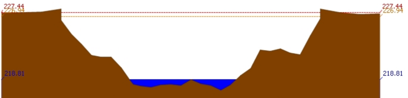
สถานี 070113T แม่น้ำวังที่ จ.ลำปาง ต.เวียงเหนือ อ.เมืองลำปาง จ.ลำปาง ระดับน้ำ 218.81 ม.รทก.
