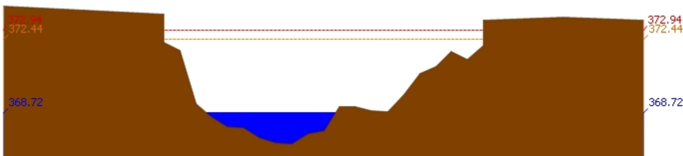
สถานี 060109T แม่น้ำปิงที่บ้านสบอ้อ ต.แม่ปะ อ.เชียงดาว จ.เชียงใหม่ ระดับน้ำ 368.72 ม.รทก.
