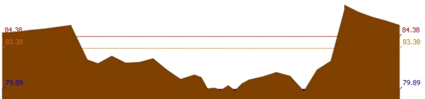
สถานี 062001T คลองสวนหมากที่บ้านน้ำไทรง ต.ท่าขุนราม อ.เมือง จ.กำแพงเพชร ระดับน้ำ 79.89 ม.รทก.
