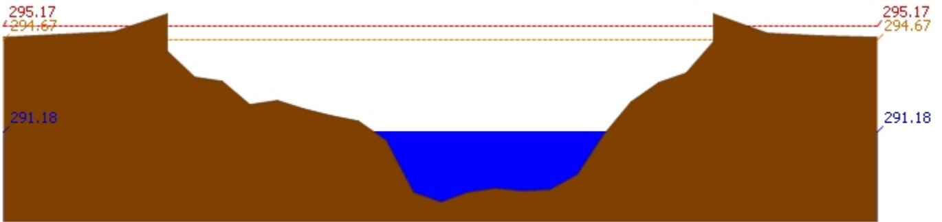
สถานี 060709T น้ำแม่กวังที่ลำพูน ต.เวียงของ อ.เมือง จ.ลำพูน ระดับน้ำ 291.18 ม.รทก.
