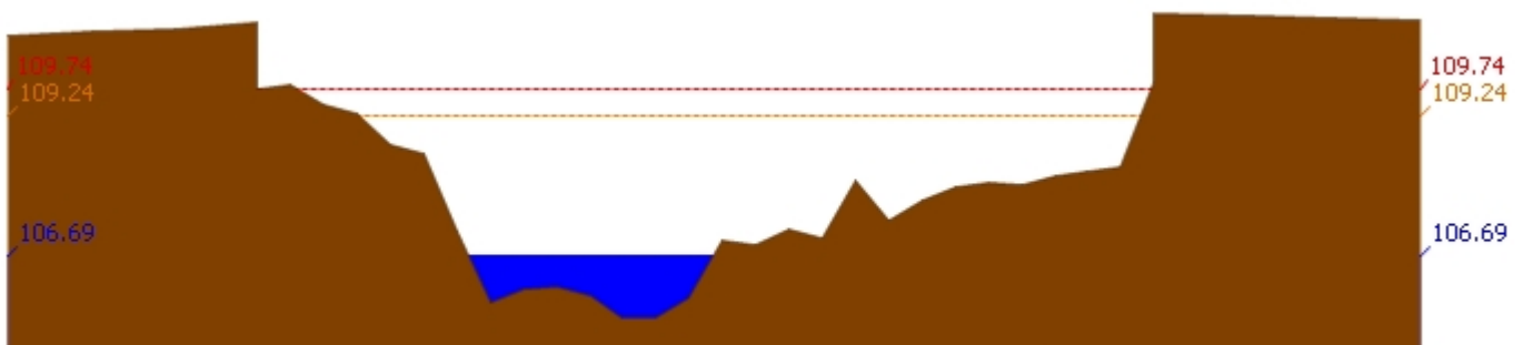
สถานี 061701T ห้วยแม่ท้อที่อำเภอเมืองตาก ต.แม่ท้อ อ.เมืองตาก จ.ตาก ระดับน้ำ 106.69 ม.รทก.
