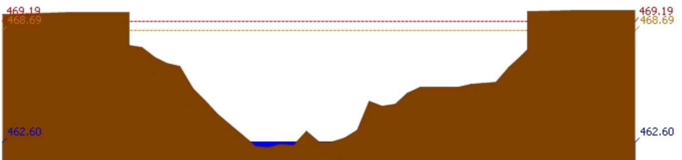
สถานี 060905T น้ำแม่ลี้ที่อำเภอลี้ ต.ลี้ อ.ลี้ จ.ลำพูน ระดับน้ำ 462.60 ม.รทก.
