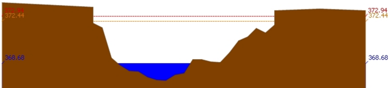
สถานี 060109T แม่น้ำปิงที่บ้านสบอ้อ ต.แม่ทะ อ.เชียงดาว จ.เชียงใหม่ ระดับน้ำ 368.68 ม.รทก.
