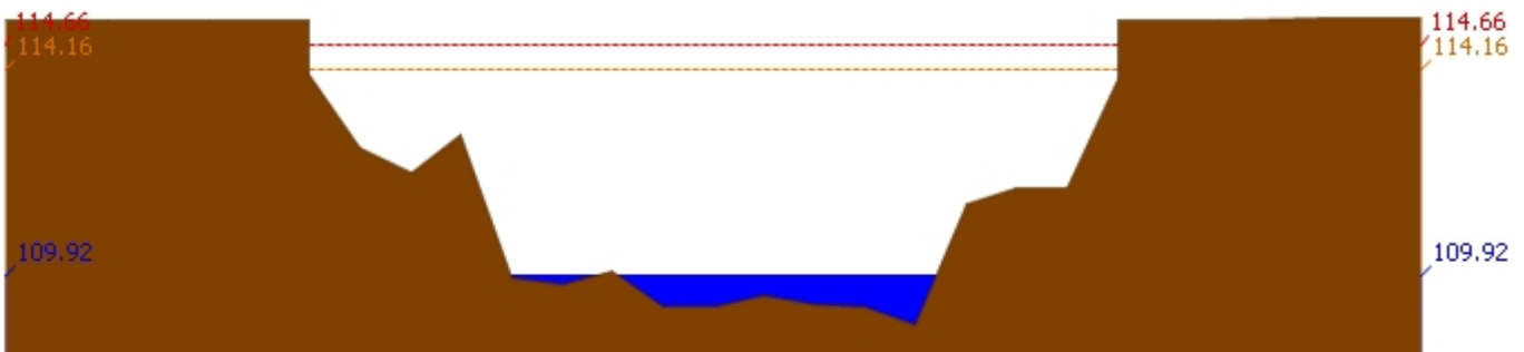
สถานี 061801T คลองวังเจ้าที่บ้านคลองลึก ต.เชียงทอง อ.วังเจ้า จ.ตาก ระดับน้ำ 109.92 ม.รทก.
