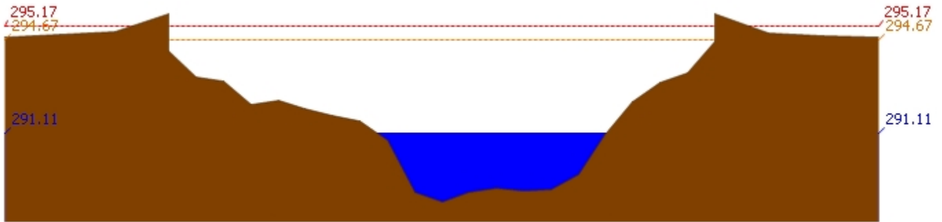
สถานี 060709T น้ำแม่กวังที่ลำพูน ต.เวียงของ อ.เมือง จ.ลำพูน ระดับน้ำ 291.11 ม.รทก.
