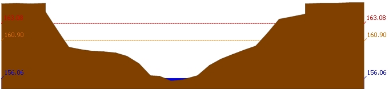
สถานี 120105T แม่น้ำป่าสักที่บ้านวังมเสหนือ ต.ทำอัญญ อ.หล่มสัก จ.เพชรบูรณ์ ระดับน้ำ 156.06 ม.รทก.
