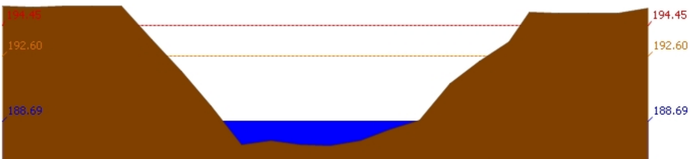
สถานี 120901T ห้วยมวกเหล็กที่ อ.มวกเหล็ก ต.มวกเหล็ก อ.มวกเหล็ก จ.สระบุรี ระดับน้ำ 188.69 ม.รทก.
