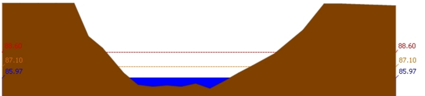
สถานี 120110T แม่น้ำป่าสักที่บ้านวังโบสถ์ ต.วังโบสถ์ อ.หนองไผ่ จ.เพชรบูรณ์ ระดับน้ำ 85.97 ม.รทก.
