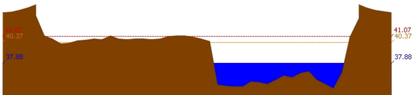
สถานี 060110T แม่น้ำปิงที่บ้านบางแก้ว ต.บางแก้ว อ.บรรพตพิสัย จ.นครสวรรค์ ระดับน้ำ 37.88 ม.รทก.
