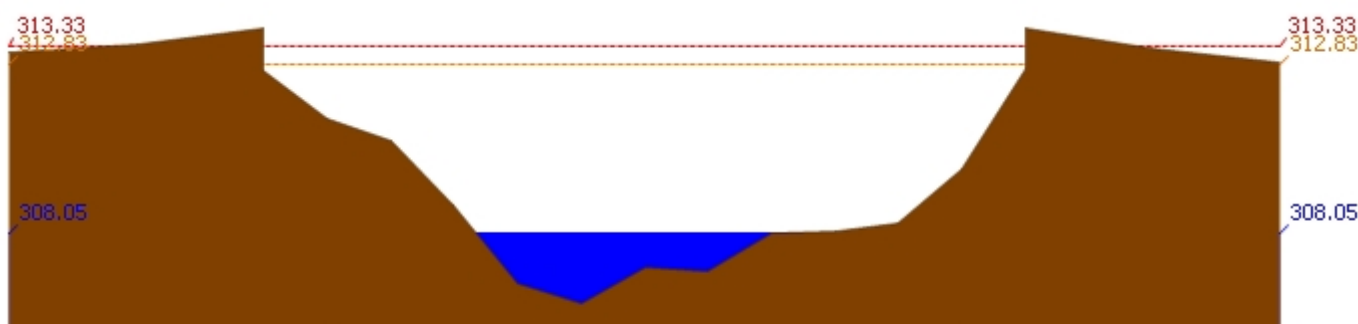
สถานี 060814T น้ำแม่ขานที่บ้านท่าโป่ง ต.บ้านแม อ.สันป่าตอง จ.เชียงใหม่ ระดับน้ำ 308.05 ม.รทก.
