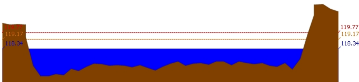
สถานี 060111T แม่น้ำปิงที่บ้านปากร่องห้วยจี้ ต.ตากออก อ.บ้านตาก จ.ตาก ระดับน้ำ 118.34 ม.รทก.
