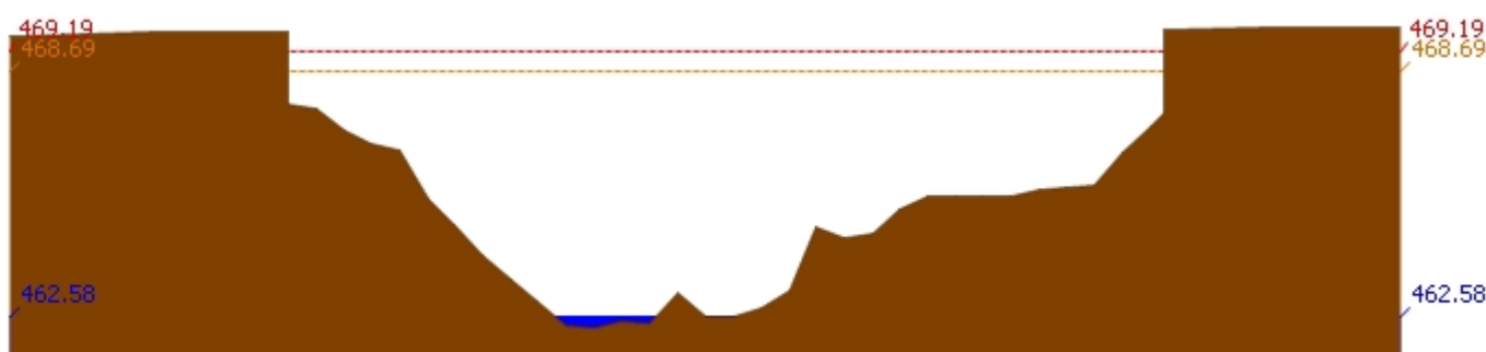
สถานี 060905T น้ำแม่ลี้ที่อำเภอลี้ ต.ลี้ อ.ลี้ จ.ลำพูน ระดับน้ำ 462.58 ม.รทก.
