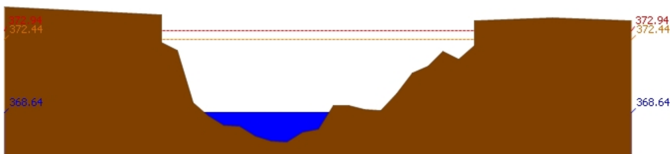
สถานี 060109T แม่น้ำปิงที่บ้านสบอ้อ ต.แม่ระ อ.เชียงดาว จ.เชียงใหม่ ระดับน้ำ 368.64 ม.รทก.
