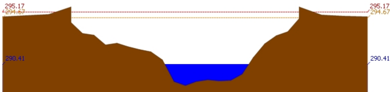
สถานี 060709T น้ำแม่กวังที่ลำพูน ต.เวียงของ อ.เมือง จ.ลำพูน ระดับน้ำ 290.41 ม.รทก.
