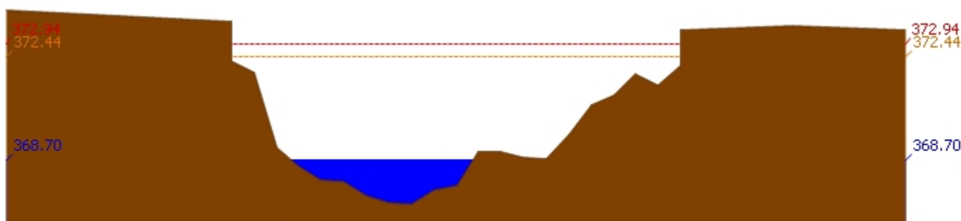
สถานี 060109T แม่น้ำปิงที่บ้านสบอ้อ ต.แม่นะ อ.เชียงดาว จ.เชียงใหม่ ระดับน้ำ 368.70 ม.รทก.
