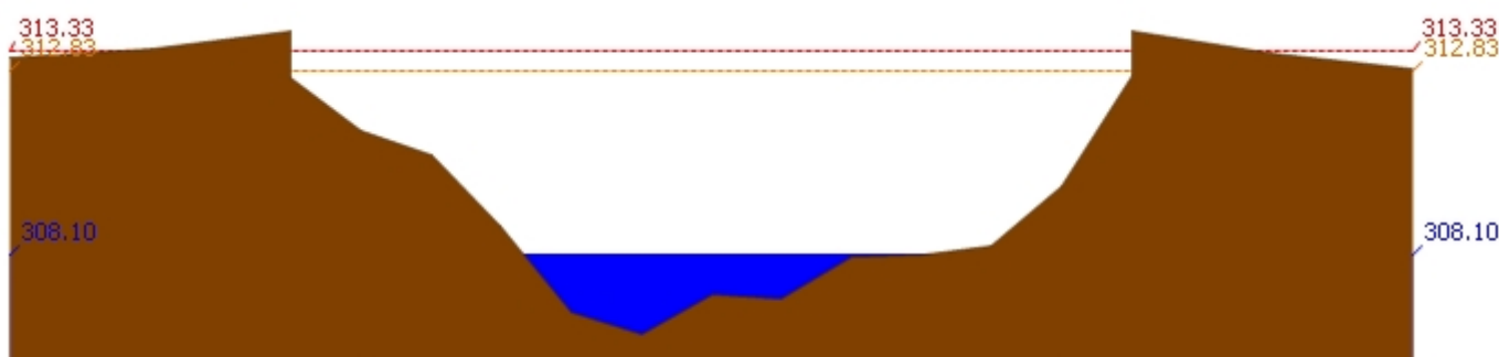
สถานี 060814T น้ำแม่ขานที่บ้านท่าโป่ง ต.บ้านแม่ อ.สันป่าตอง จ.เชียงใหม่ ระดับน้ำ 308.10 ม.รทก.
