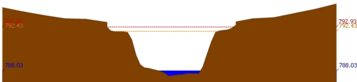
สถานี 061503T น้ำแม่ต้นที่บ้านคอย ต.ยางเปียง อ.อมก๋อย จ.เชียงใหม่ ระดับน้ำ 788.03 ม.รทก.
