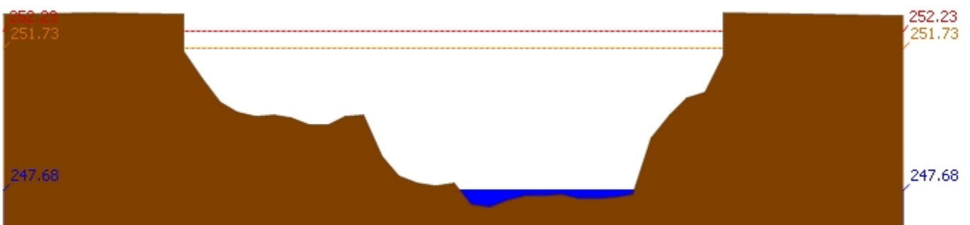
สถานี 070403T น้ำแม่ตุ๋ยที่บ้านแค ต.บ้านเป้า อ.เมืองลำปาง จ.ลำปาง ระดับน้ำ 247.68 ม.รทก.
