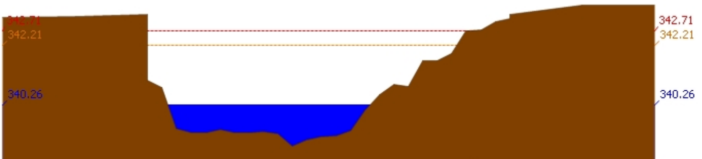
สถานี 070304T น้ำแม่สอยที่บ้านหนองกอก ต.แม่สุก อ.แจ้ห่ม จ.ลำปาง ระดับน้ำ 340.26 ม.รทก.
