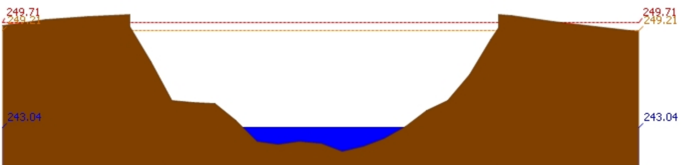
สถานี 070112T แม่น้ำวังที่บ้านบุญนาค ต.บุญนาคพัฒนา อ.เมืองลำปาง จ.ลำปาง ระดับน้ำ 243.04 ม.รทก.
