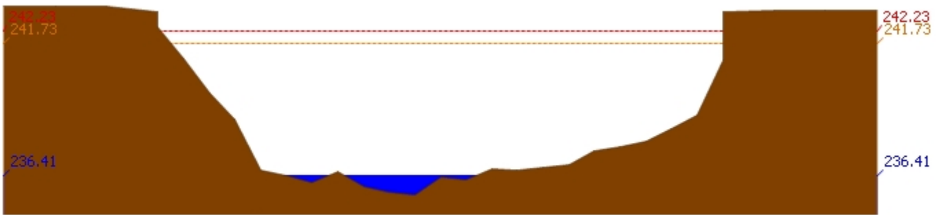
สถานี 070114T แม่น้ำวังที่บ้านปางชัย ต.บ้านเสด็จ อ.เมืองลำปาง จ.ลำปาง ระดับน้ำ 236.41 ม.รทก.
