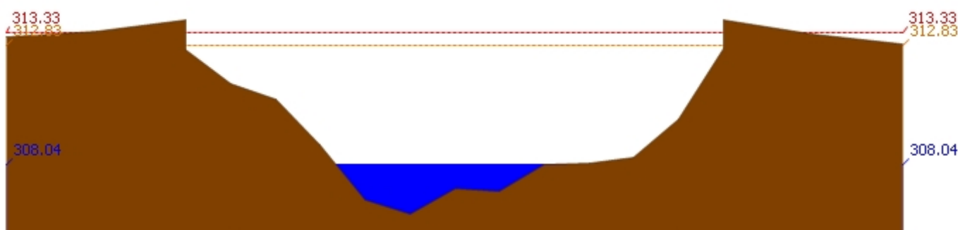
สถานี 060814T น้ำแม่ขานที่บ้านท่าโป่ง ต.บ้านแม อ.สันป่าตอง จ.เชียงใหม่ ระดับน้ำ 308.04 ม.รทก.
