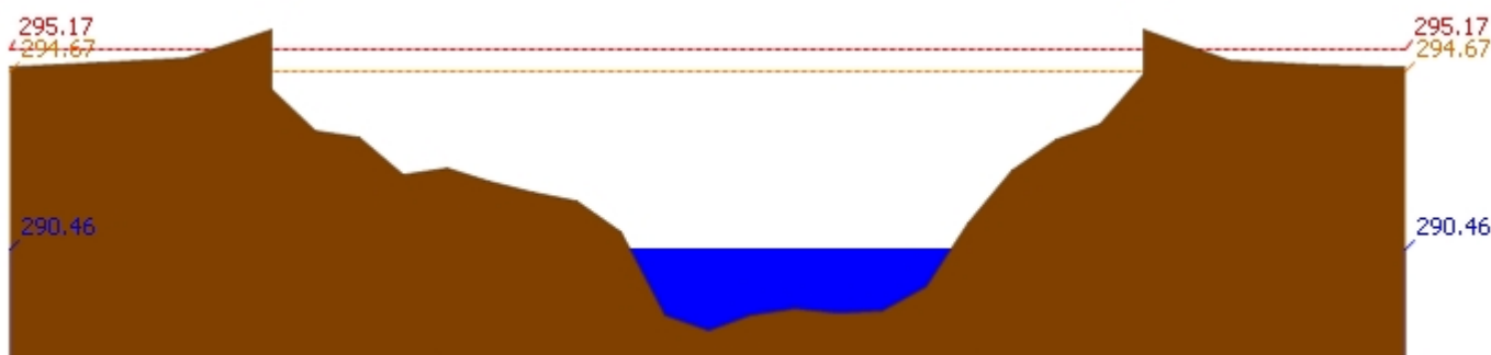
สถานี 060709T น้ำแม่กวังที่ลำพูน ต.เวียงของ อ.เมือง จ.ลำพูน ระดับน้ำ 290.46 ม.รทก.
