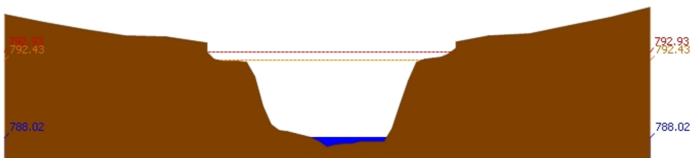
สถานี 061503T น้ำแม่ต้นที่บ้านคอย ต.ยางเปียง อ.อมก๋อย จ.เชียงใหม่ ระดับน้ำ 788.02 ม.รทก.
