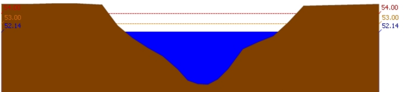
สถานี 120702T ลำสนธิที่บ้านท่าช้าง ต.หนองขาหย่าง อ.ชัยบาดาล จ.ลพบุรี ระดับน้ำ 52.14 ม.รทก.
