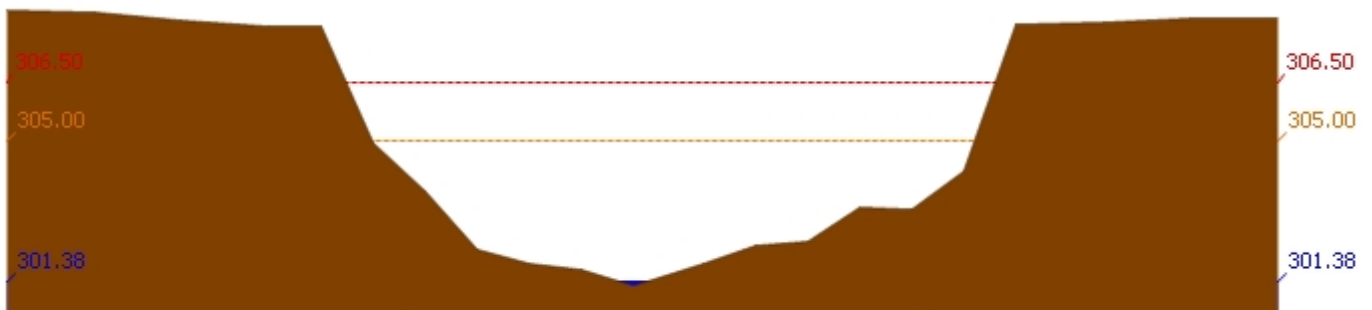
สถานี 120304T หัวน้ำพุที่บ้านกกกะบาก ต.โป่ง อ.ด่านซ้าย จ.เลย ระดับน้ำ 301.38 ม.รทก.
