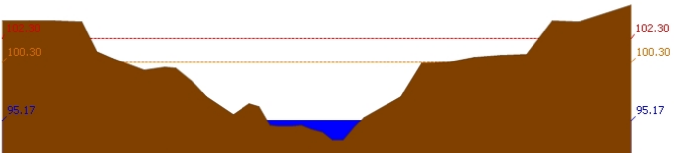
สถานี 120112T แม่น้ำป่าสักที่บ้านหนองแหวน ต.วังมะข่อ อ.เมือง จ.เพชรบูรณ์ ระดับน้ำ 95.17 ม.รทก.
