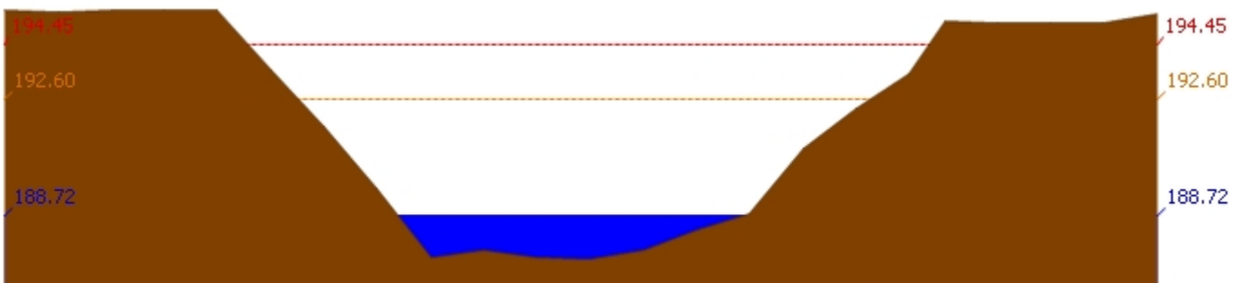
สถานี 120901T ฝายมวกเหล็กที่ อ.มวกเหล็ก ต.มวกเหล็ก อ.มวกเหล็ก จ.สระบุรี ระดับน้ำ 188.72 ม.รทก.
