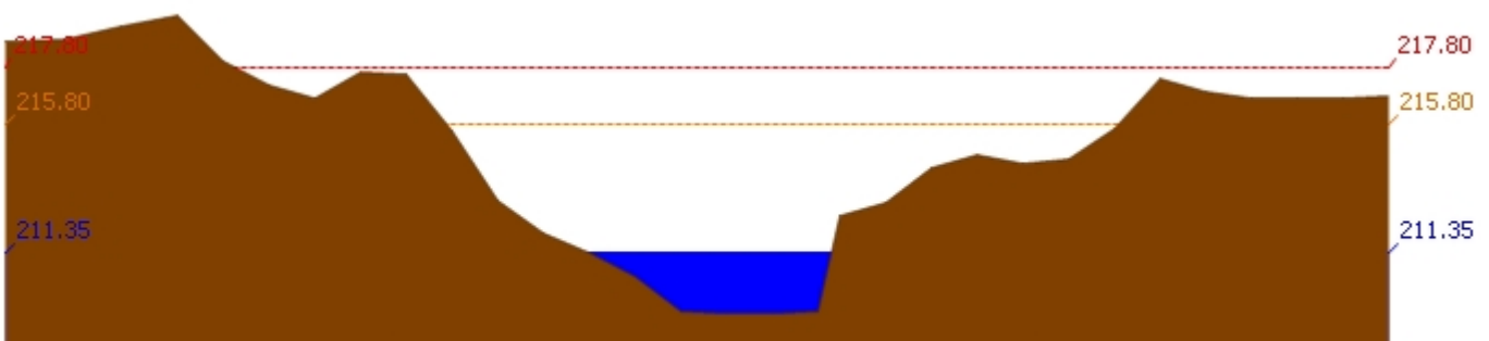
สถานี 120205T แม่น้ำป่าสักที่บ้านอุมกะทาด ต.ศิลา อ.หล่มเก่า จ.เพชรบูรณ์ ระดับน้ำ 211.35 ม.รทก.
