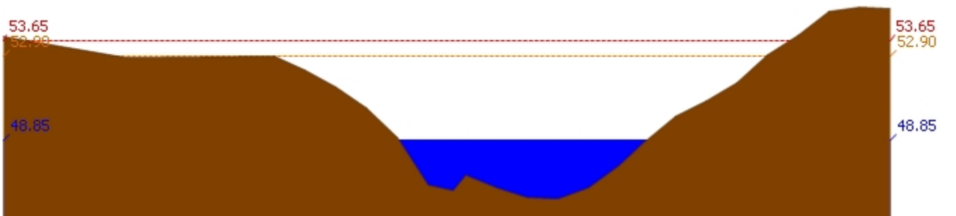
สถานี 120113T แม่น้ำป่าสักที่บ้านเขาค้าง ต.คลองกระจิง อ.ศรีเทพ จ.เพชรบูรณ์ ระดับน้ำ 48.85 ม.รทก.
