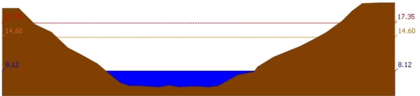
สถานี 120109T แม่น้ำป่าสักที่ อ.แก่งคอย ต.แก่งคอย อ.แก่งคอย จ.สระบุรี ระดับน้ำ 8.12 ม.รทก.
