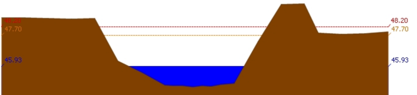
สถานี 110303T คลองโพธิ์ที่บ้านทุ่งสงบ ต.ไม้เขี้ยว อ.สว่างอารมณ์ จ.อุทัยธานี ระดับน้ำ 45.93 ม.รทก.
