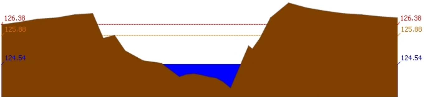
สถานี 110301T คลองโพธิ์ที่บ้านคลองบัวสามัคคี ต.ปางสวรรค์ อ.ชุมตาบง จ.นครสวรรค์ ระดับน้ำ 124.54 ม.รทก.
