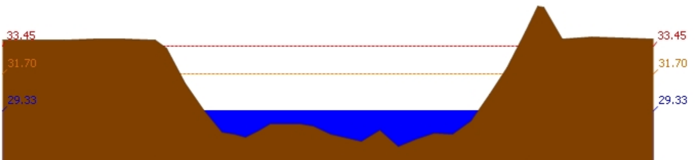
สถานี 110503T แม่น้ำตากแดดที่บ้านหนองขาลาย ต.หนองหลวง อ.สว่างอารมณ์ จ.อุทัยธานี ระดับน้ำ 29.33 ม.รทก.
