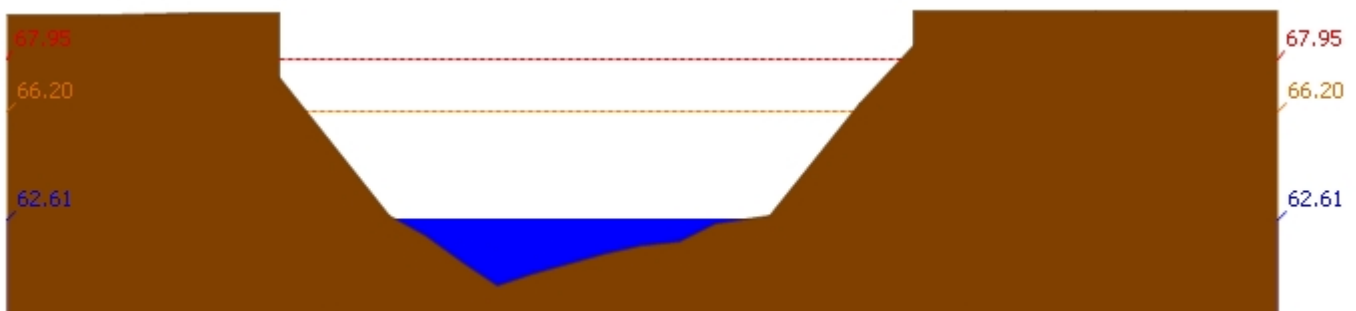
สถานี 110501T น้ำแม่วังที่บ้านคลองสาลี ต.ลาดยาว อ.ลาดยาว จ.นครสวรรค์ ระดับน้ำ 62.61 ม.รทก.
