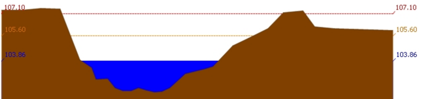
สถานี 110402T ห้วยทับเสลาที่บ้านนาไร่เดียว ต.ลานสัก อ.ลานสัก จ.อุทัยธานี ระดับน้ำ 103.86 ม.รทก.
