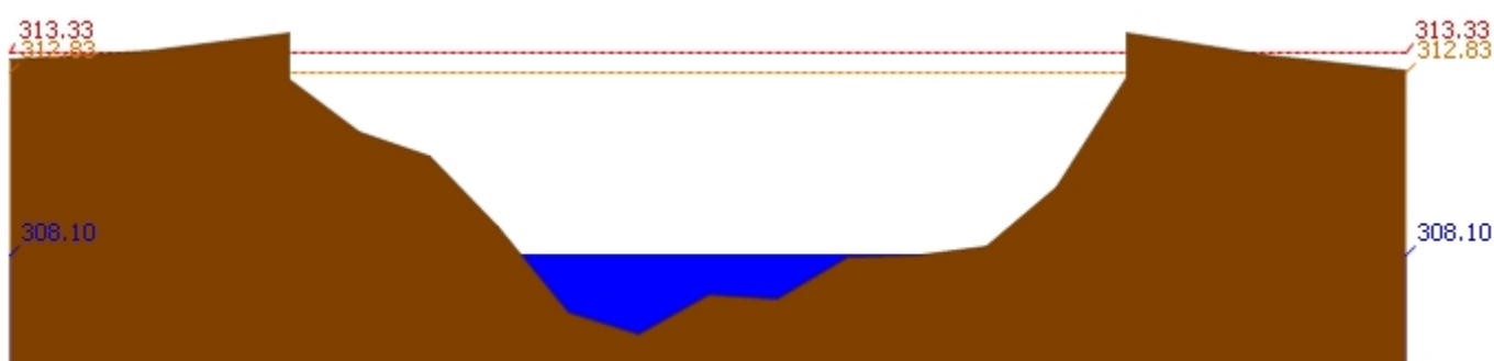
สถานี 060814T น้ำแม่ขานที่บ้านท่าโป่ง ต.บ้านแม อ.สันป่าตอง จ.เชียงใหม่ ระดับน้ำ 308.10 ม.รทก.
