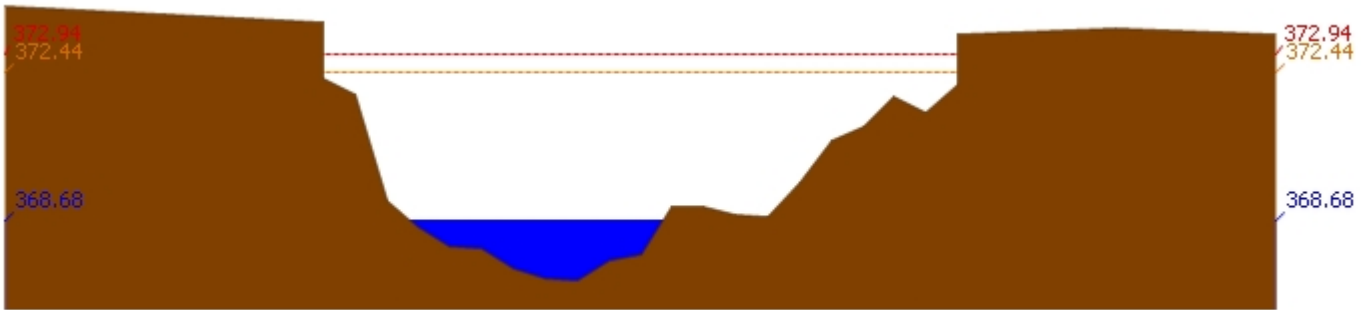
สถานี 060109T แม่น้ำปิงที่บ้านสบอ้อ ต.แม่ระ อ.เชียงดาว จ.เชียงใหม่ ระดับน้ำ 368.68 ม.รทก.
