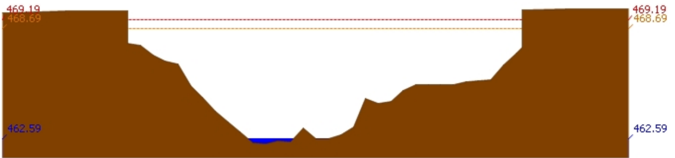
สถานี 060905T น้ำแม่ลี้ที่อำเภอลี้ ต.ลี้ อ.ลี้ จ.ลำพูน ระดับน้ำ 462.59 ม.รทก.
