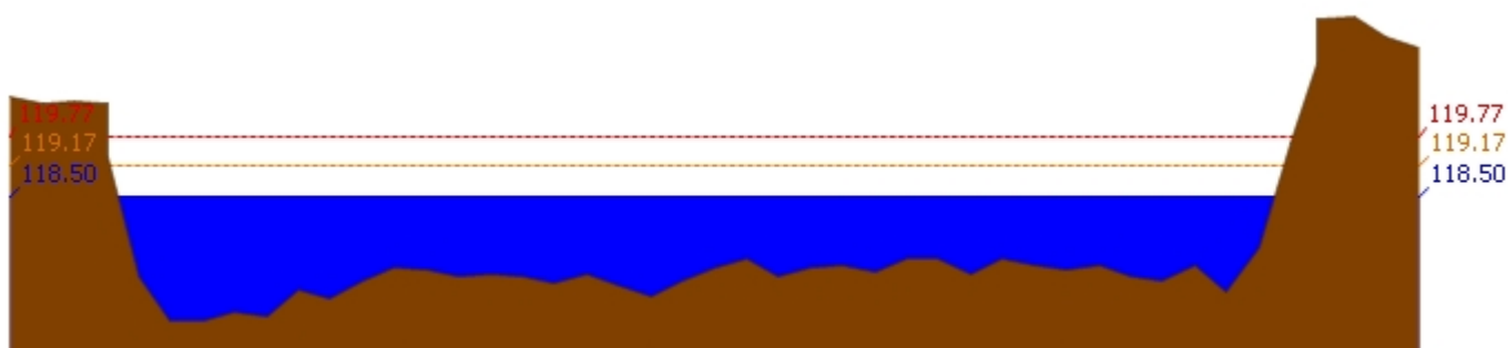
สถานี 060111T แม่น้ำปิงที่บ้านปากร่องห้วยจี่ ต.ตากออก อ.บ้านตาก จ.ตาก ระดับน้ำ 118.50 ม.รทก.
