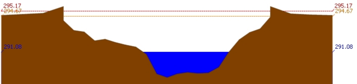
สถานี 060709T น้ำแม่กวงที่ลำพูน ต.เวียงของ อ.เมือง จ.ลำพูน ระดับน้ำ 291.08 ม.รทก.
