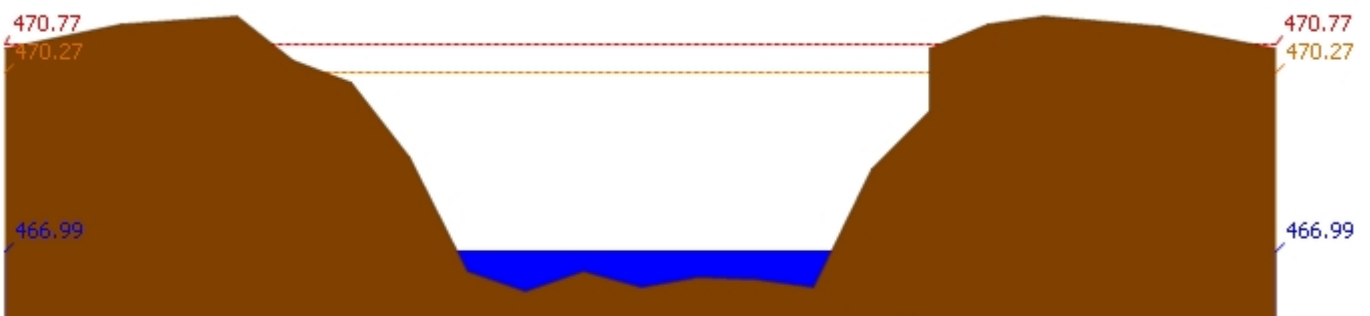
สถานี 061206T น้ำแม่แจ่มที่บ้านทัพ ต.ท่าผา อ.แม่แจ่ม จ.เชียงใหม่ ระดับน้ำ 466.99 ม.รทก.
