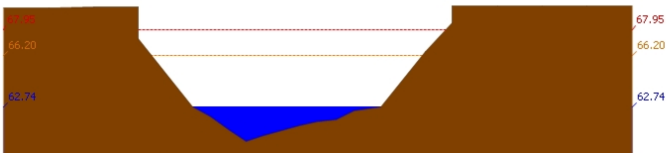
สถานี 110501T น้ำแมวกักที่บ้านคลองสาลี ต.ลาดยาว อ.ลาดยาว จ.นครสวรรค์ ระดับน้ำ 62.74 ม.รทก.
