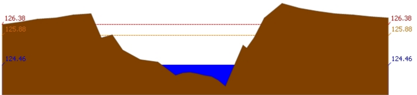
สถานี 110301T คลองโพธิ์ที่บ้านคลองบัวสามัคคี ต.ปางสวรรค์ อ.ชุมตาบง จ.นครสวรรค์ ระดับน้ำ 124.46 ม.รทก.
