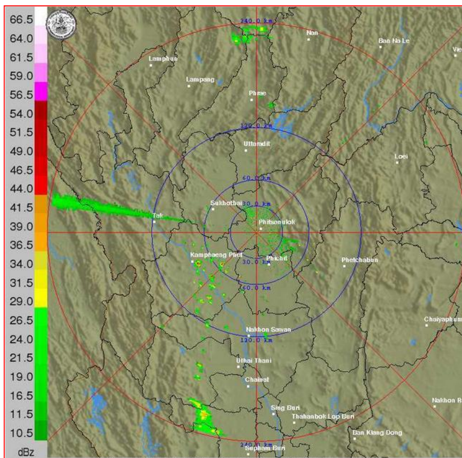
ภาพเรดาร์ตรวจอากาศ “พิษณุโลก” ณ วันที่ 1 พฤษภาคม 2561 (ที่มา : กรมอุตุนิยมวิทยา)
