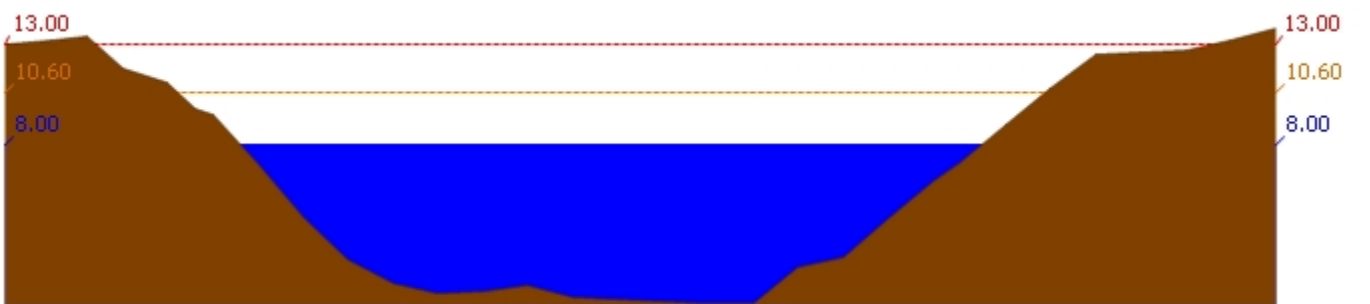
สถานี 120106T แม่น้ำป่าสักที่ อ.เสาไห้ ต.ศาลาวิไทย อ.เสาไห้ จ.สระบุรี ระดับน้ำ 8.00 ม.รทก.
