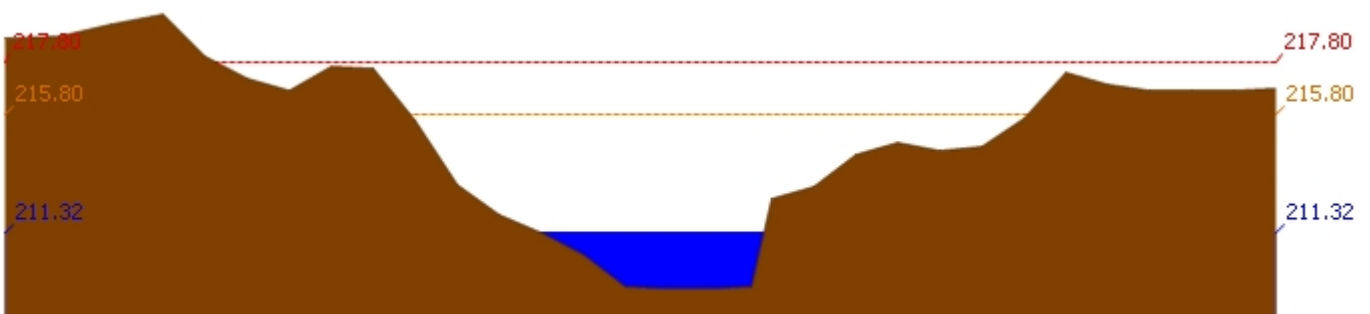
สถานี 120205T แม่น้ำป่าสักที่บ้านอุมกะทาด ต.ศิลา อ.หล่มเก่า จ.เพชรบูรณ์ ระดับน้ำ 211.32 ม.รทก.
