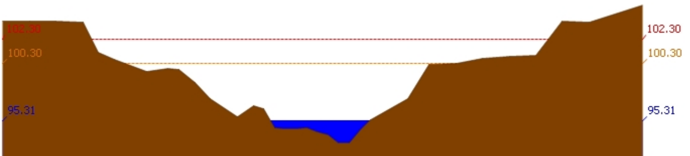
สถานี 120112T แม่น้ำป่าสักที่บ้านหนองแหวน ต.วังมะข่อ อ.เมือง จ.เพชรบูรณ์ ระดับน้ำ 95.31 ม.รทก.
