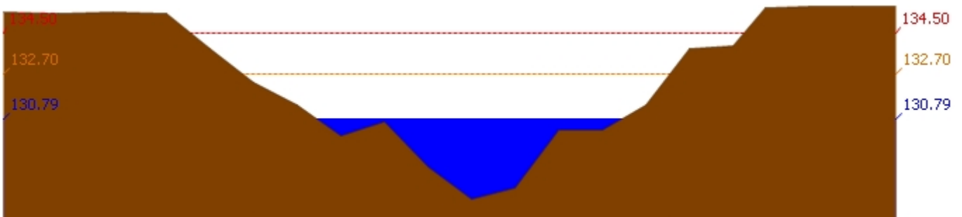
สถานี 120111T แม่น้ำป่าสักที่บ้านจางวาง ต.ลานบ่า อ.หล่มสัก จ.เพชรบูรณ์ ระดับน้ำ 130.79 ม.รทก.
