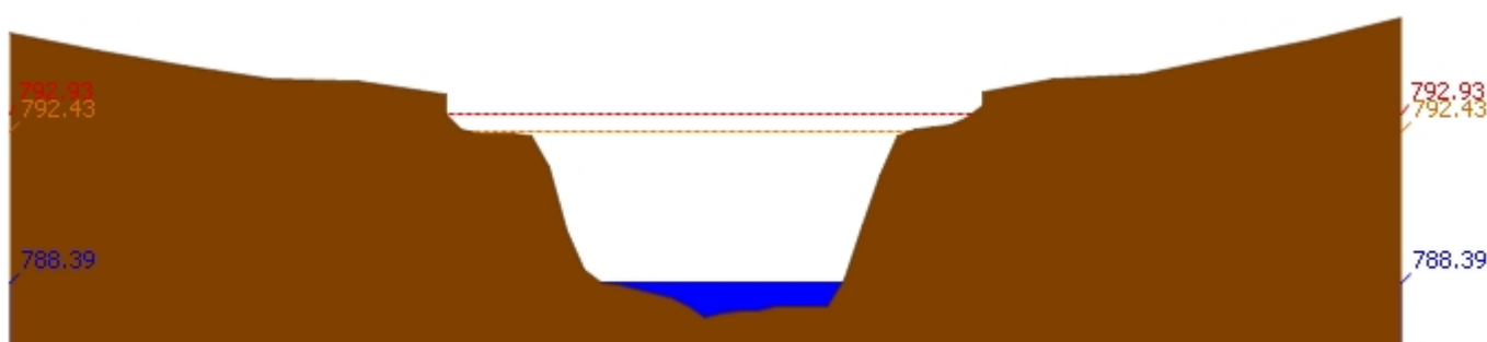
สถานี 061503T น้ำแม่ต้นที่บ้านคอย ต.ยางเปียง อ.อมก๋อย จ.เชียงใหม่ ระดับน้ำ 788.39 ม.รทก.
