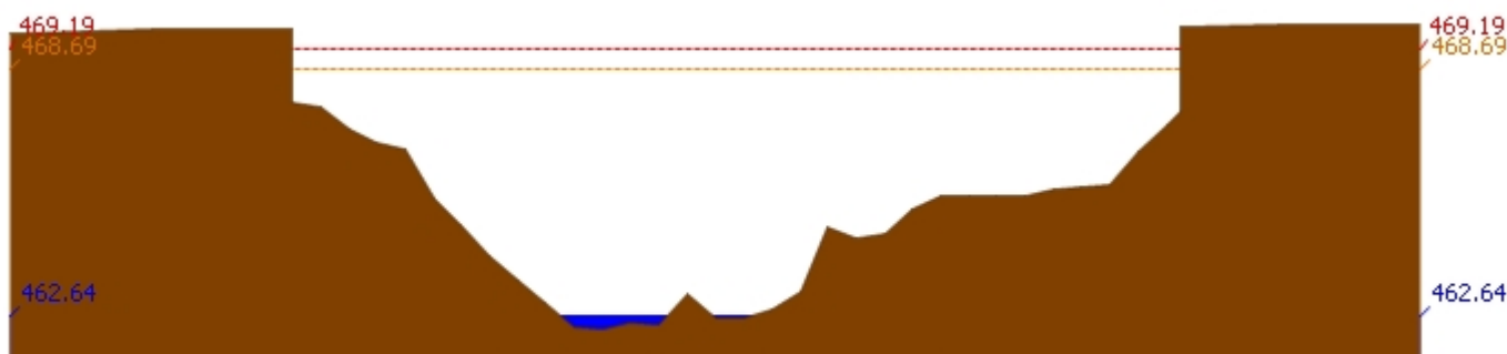
สถานี 060905T น้ำแม่สีที่อำเภอสีคิ้ว อ.สีคิ้ว จ.ลำพูน ระดับน้ำ 462.64 ม.รทก.
