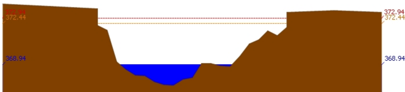
สถานี 060109T แม่น้ำปิงที่บ้านสบฮ้อ ต.แม่ระ อ.เชียงดาว จ.เชียงใหม่ ระดับน้ำ 368.94 ม.รทก.
