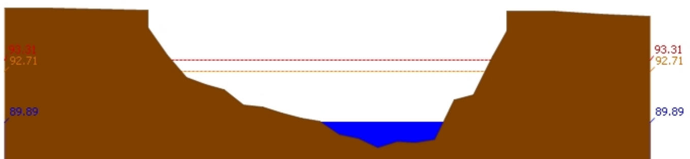
สถานี 061901T คลองแม่ระกาที่บ้านวังชะโอน ต.ท่าไม้ อ.พราหมณ์ จ.กำแพงเพชร ระดับน้ำ 89.89 ม.รทก.
