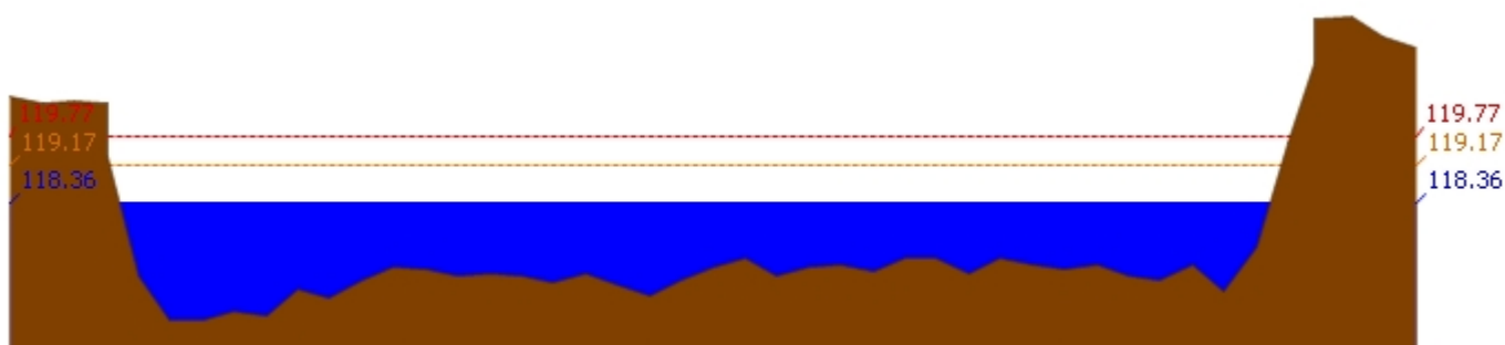
สถานี 060111T แม่น้ำปิงที่บ้านปากร่องห้วยจี้ ต.ตากออก อ.บ้านตาก จ.ตาก ระดับน้ำ 118.36 ม.รทก.
