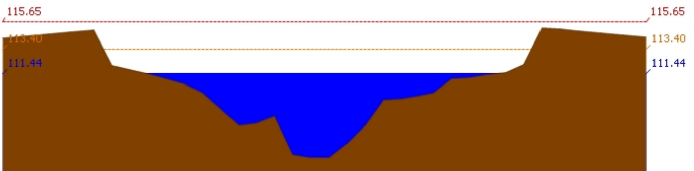
สถานี 120107T แม่น้ำป่าสักที่ อ.เมืองเพชรบูรณ์ ต.นาป่า อ.เมือง จ.เพชรบูรณ์ ระดับน้ำ 111.44 ม.รทก.
