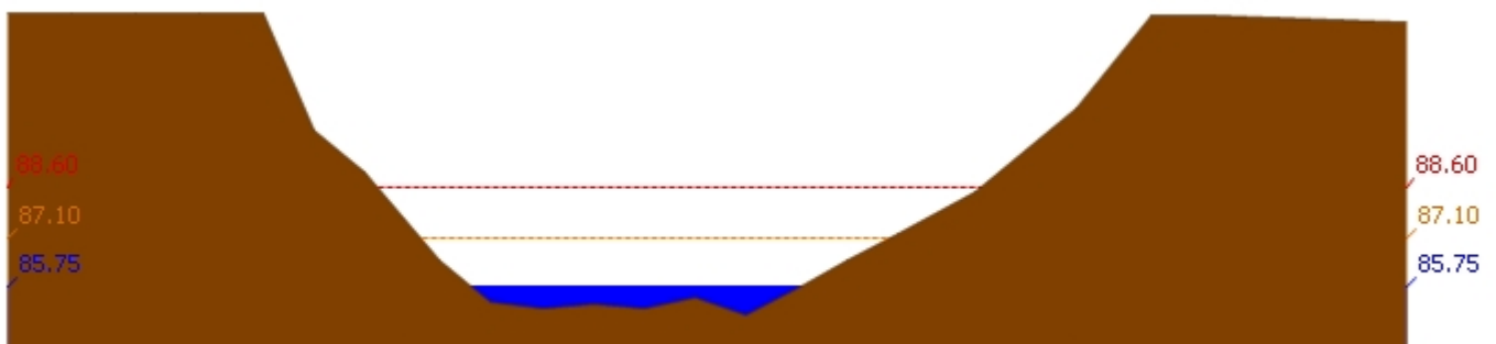
สถานี 120110T แม่น้ำป่าสักที่บ้านวังโบสถ์ ต.วังโบสถ์ อ.หนองไผ่ จ.เพชรบูรณ์ ระดับน้ำ 85.75 ม.รทก.
