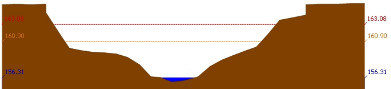
สถานี 120105T แม่น้ำป่าสักที่บ้านวังมลเหนือ ต.ทำอัญญ อ.หล่มสัก จ.เพชรบูรณ์ ระดับน้ำ 156.31 ม.รทก.
