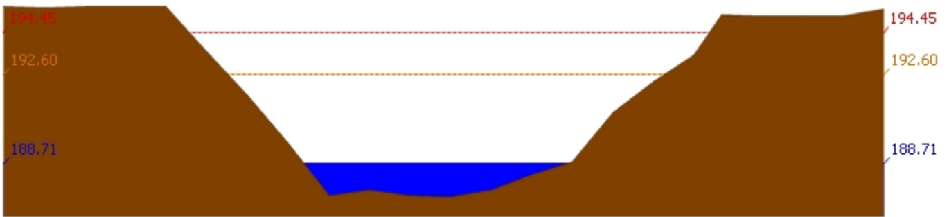
สถานี 120901T ฝั้วยมวกเหล็กที่ อ.มวกเหล็ก ต.มวกเหล็ก อ.มวกเหล็ก จ.สระบุรี ระดับน้ำ 188.71 ม.รทก.
