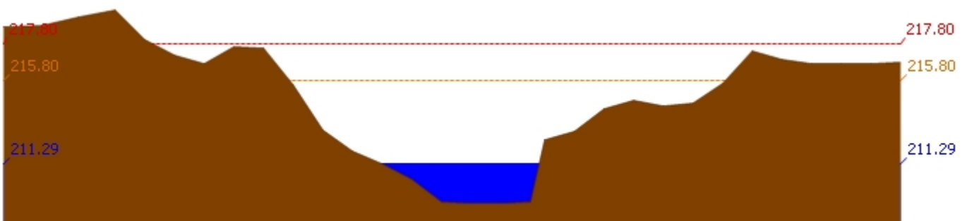
สถานี 120205T แม่น้ำป่าสักที่บ้านอุมกะทาด ต.ศิลา อ.หล่มเก่า จ.เพชรบูรณ์ ระดับน้ำ 211.29 ม.รทก.
