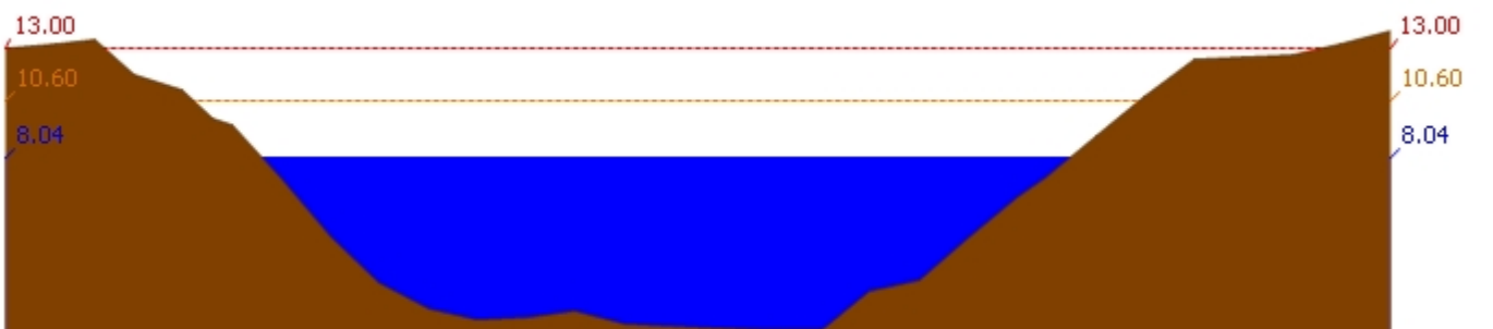
สถานี 120106T แม่น้ำป่าสักที่ อ.เสาไห้ ต.ศาลาวิไทย อ.เสาไห้ จ.สระบุรี ระดับน้ำ 8.04 ม.รทก.
