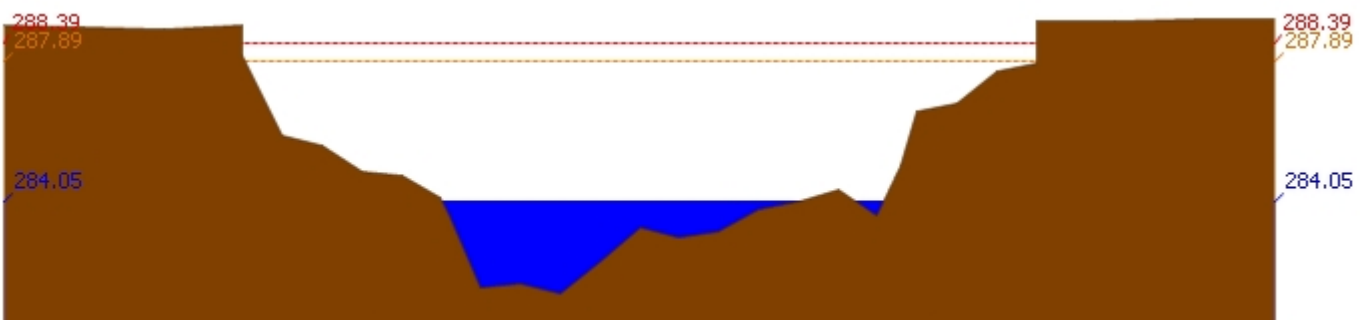
สถานี 070111T แม่บ้านวังที่บ้านแปงโปงชัย ต.บ้านเสา อ.แจ้ห่ม จ.ลำปาง ระดับน้ำ 284.05 ม.รทก.
