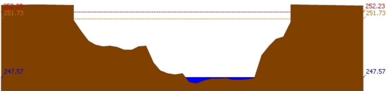
สถานี 070403T น้ำแม่คู่ที่บ้านแค้ ต.บ้านเป้า อ.เมืองลำปาง จ.ลำปาง ระดับน้ำ 247.57 ม.รทก.
