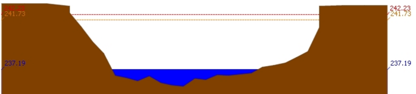
สถานี 070114T แม่น้ำวังที่บ้านปงชัย ต.บ้านเสด็จ อ.เมืองลำปาง จ.ลำปาง ระดับน้ำ 237.19 ม.รทก.
