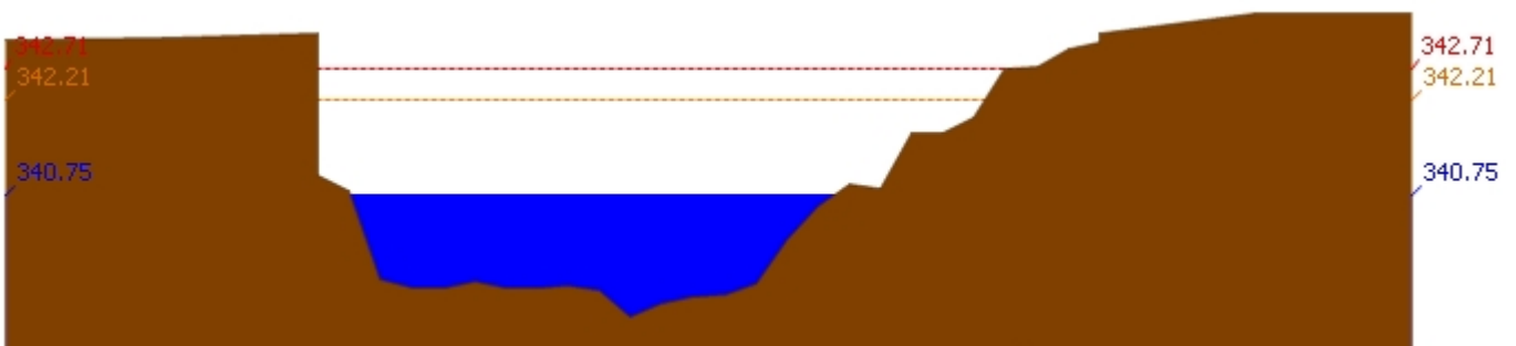
สถานี 070304T น้ำแม่สอยที่บ้านหนองกอก ต.แม่สุก อ.แจ้ห่ม จ.ลำปาง ระดับน้ำ 340.75 ม.รทก.
