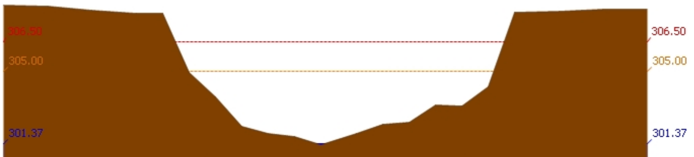
สถานี 120304T หัวน้ำพุที่บ้านกกกะบาก ต.โป่ง อ.ด่านซ้าย จ.เลย ระดับน้ำ 301.37 ม.รทก.
