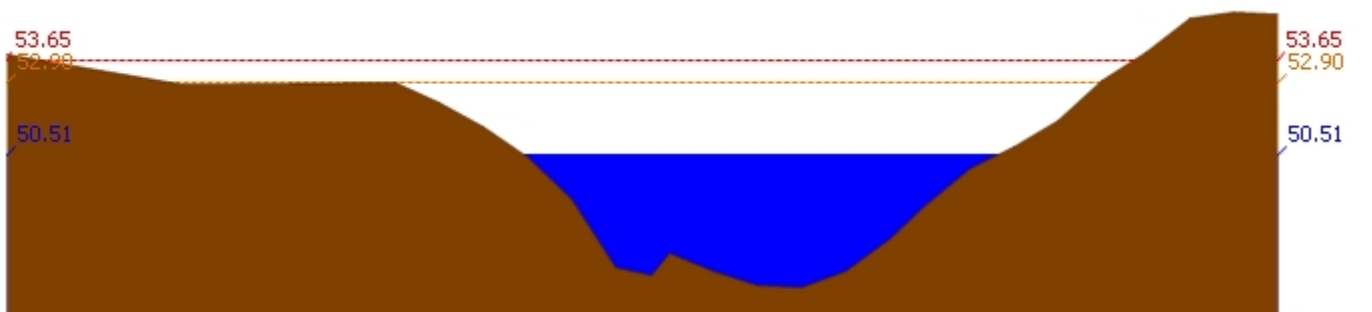
สถานี 120113T แม่น้ำป่าสักที่บ้านเขาค้าง ต.คลองกระจิง อ.ศรีเทพ จ.เพชรบูรณ์ ระดับน้ำ 50.51 ม.รทก.
