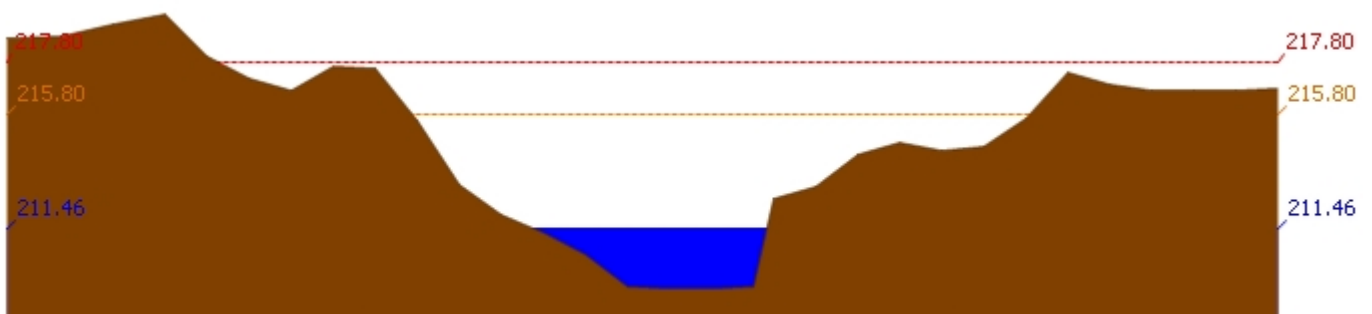
สถานี 120205T แม่น้ำป่าสักที่บ้านอุมกะทาด ต.ศิลา อ.หล่มเก่า จ.เพชรบูรณ์ ระดับน้ำ 211.46 ม.รทก.
