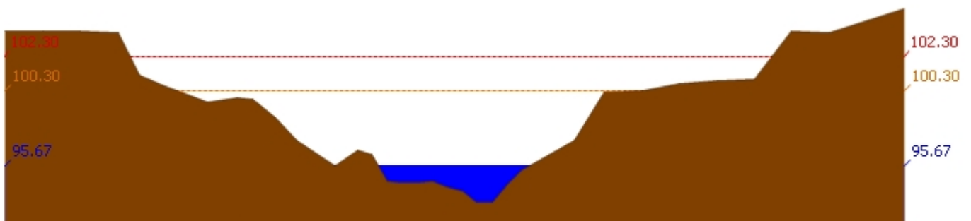
สถานี 120112T แม่น้ำป่าสักที่บ้านหนองแหวน ต.วังมะข่อ อ.เมือง จ.เพชรบูรณ์ ระดับน้ำ 95.67 ม.รทก.
