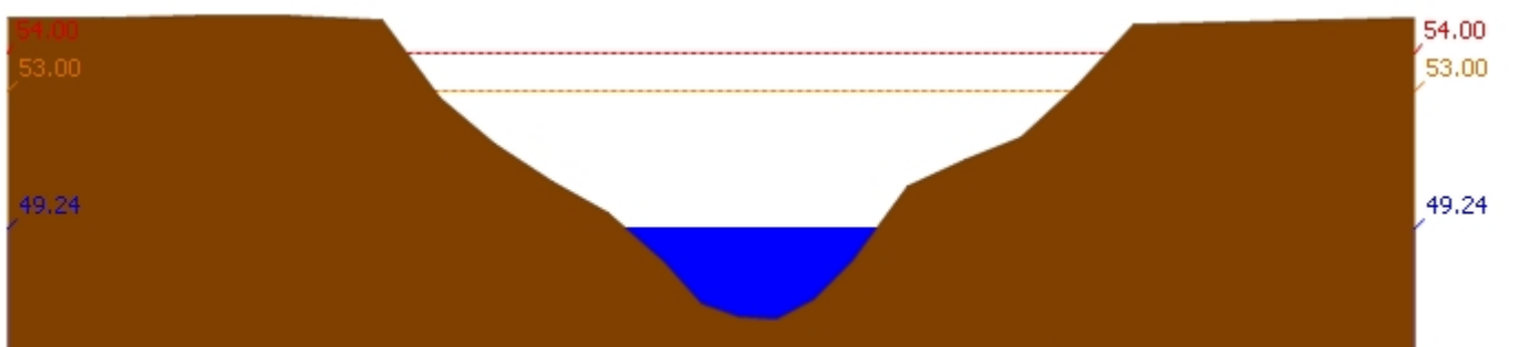
สถานี 120702T ลำสนธิที่บ้านท่าช้าง ต.หนองขาหย่าง อ.ชัยบาดาล จ.ลพบุรี ระดับน้ำ 49.24 ม.รทก.
