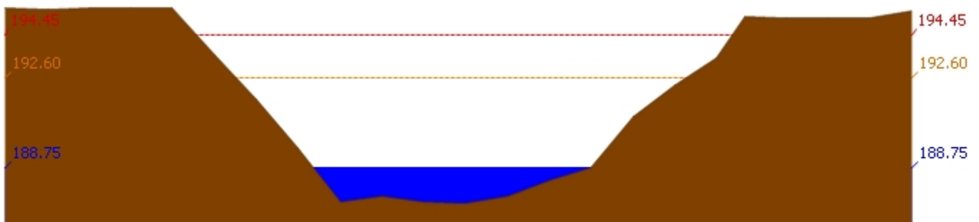
สถานี 120901T ฝั้วยมวกเหล็กที่ อ.มวกเหล็ก ต.มวกเหล็ก อ.มวกเหล็ก จ.สระบุรี ระดับน้ำ 188.75 ม.รทก.
