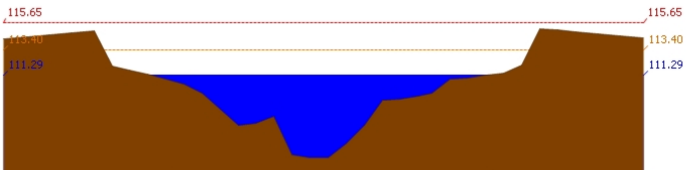
สถานี 120107T แม่น้ำป่าสักที่ อ.เมืองเพชรบูรณ์ ต.นาป่า อ.เมือง จ.เพชรบูรณ์ ระดับน้ำ 111.29 ม.รทก.
