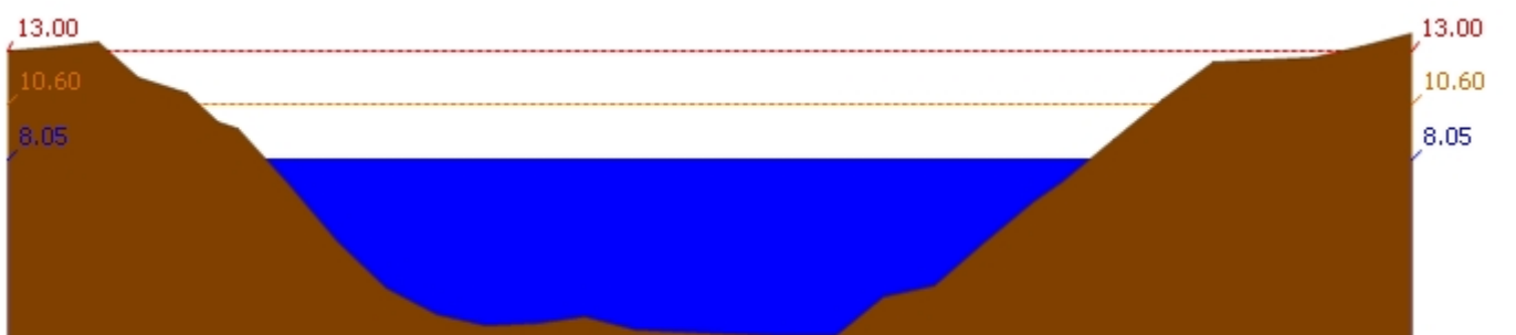
สถานี 120106T แม่น้ำป่าสักที่ อ.เสนาห์ ต.ศาลาวิไทย อ.เสนาห์ จ.สระบุรี ระดับน้ำ 8.05 ม.รทก.
