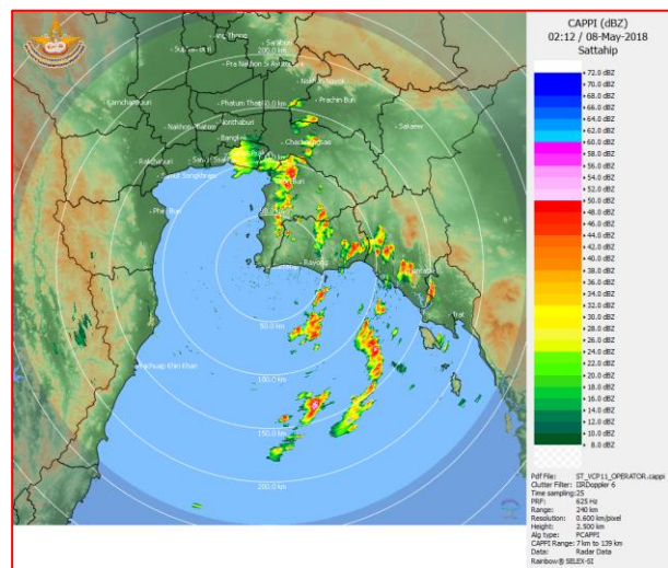
ภาพเรดาร์ตรวจอากาศ “สถานีสัตหีบ” ณ วันที่ 8 พฤษภาคม 2561 เวลา 09.12 น. (ที่มา :กรมอุตุนิยมวิทยา)
