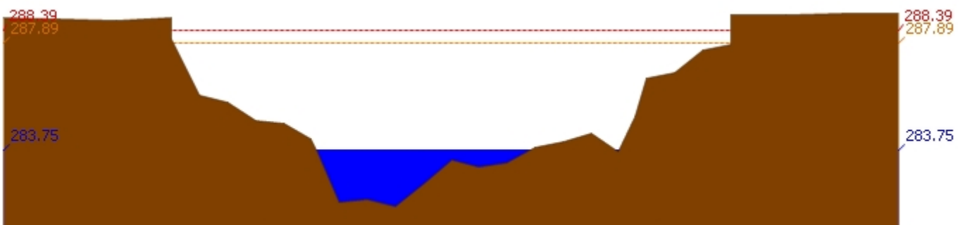
สถานี 070111T แม่บ้านวังที่บ้านแปงโปงชัย ต.บ้านเสา อ.แจ้ห่ม จ.ลำปาง ระดับน้ำ 283.75 ม.รทก.
