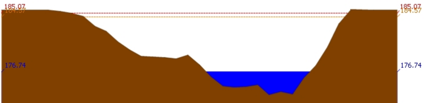
สถานี 070116T แม่น้ำวังที่บ้านแม่เตี๊ยะ ต.แม่ถอด อ.เถิน จ.ลำปาง ระดับน้ำ 176.74 ม.รทก.
