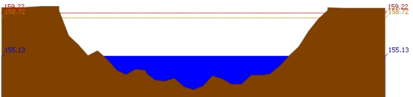
สถานี 070117T แม่น้ำวังที่เทศบาลตำบลแม่ปู ต.แม่ปู อ.แม่พริก จ.ลำปาง ระดับน้ำ 155.13 ม.รทก.
