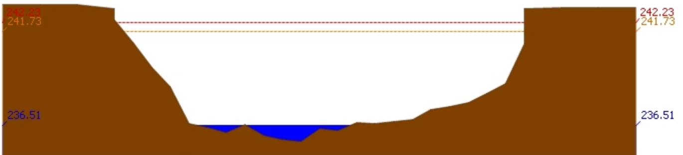
สถานี 070114T แม่น้ำวังที่บ้านปางชัย ต.บ้านเสด็จ อ.เมืองลำปาง จ.ลำปาง ระดับน้ำ 236.51 ม.รทก.
