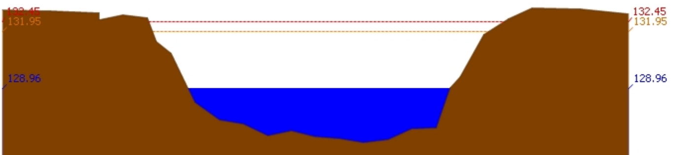
สถานี 070118T แม่น้ำวังที่บ้านแม่สลิด ต.แม่สลิด อ.บ้านตาก จ.ตาก ระดับน้ำ 128.96 ม.รทก.
