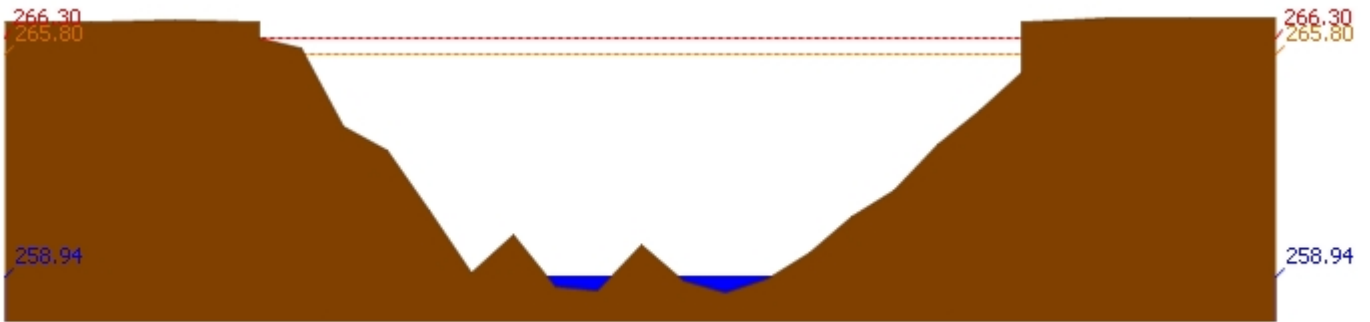
สถานี 070604T น้ำแม่จางที่บ้านสุโหมไชยมงคล ต.หัวเสือ อ.แม่ทะ จ.ลำปาง ระดับน้ำ 258.94 ม.รทก.
