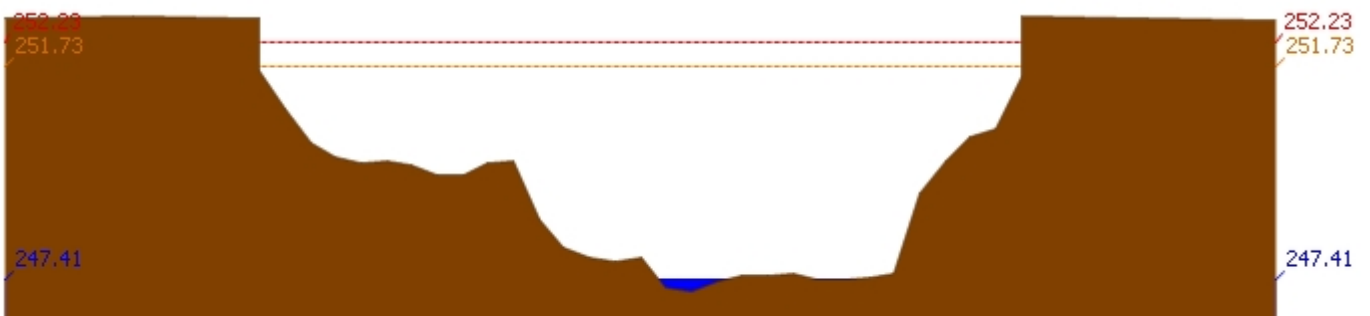
สถานี 070403T น้ำแม่คู่ที่บ้านแค้ ต.บ้านเป้า อ.เมืองลำปาง จ.ลำปาง ระดับน้ำ 247.41 ม.รทก.
