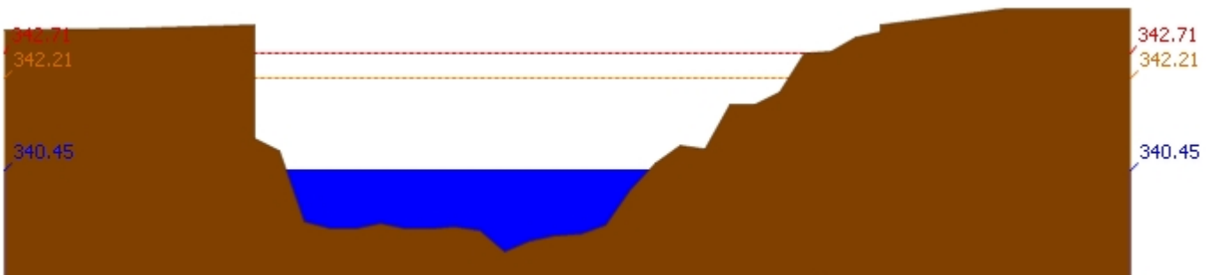
สถานี 070304T น้ำแม่สอยที่บ้านหนองกอก ต.แม่สุก อ.แจ้ห่ม จ.ลำปาง ระดับน้ำ 340.45 ม.รทก.
