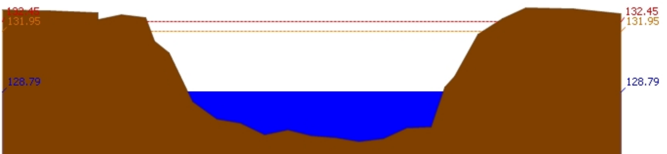
สถานี 070118T แม่น้ำวังที่บ้านแม่สลิด ต.แม่สลิด อ.บ้านตาก จ.ตาก ระดับน้ำ 128.79 ม.รทก.
