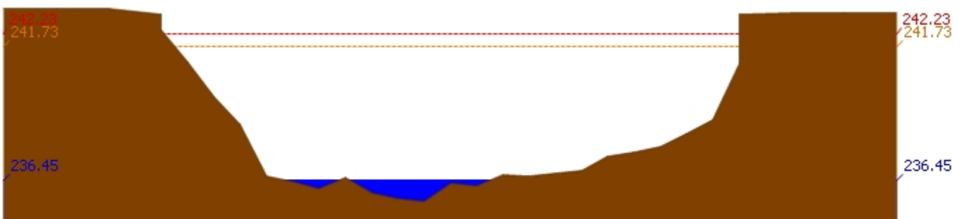
สถานี 070114T แม่น้ำวังที่บ้านปงชัย ต.บ้านเสด็จ อ.เมืองลำปาง จ.ลำปาง ระดับน้ำ 236.45 ม.รทก.
