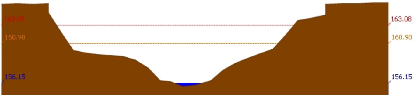
สถานี 120105T แม่น้ำป่าสักที่บ้านวังมเสเหนือ ต.ทำอัญญา อ.หล่มสัก จ.เพชรบูรณ์ ระดับน้ำ 156.15 ม.รทก.
