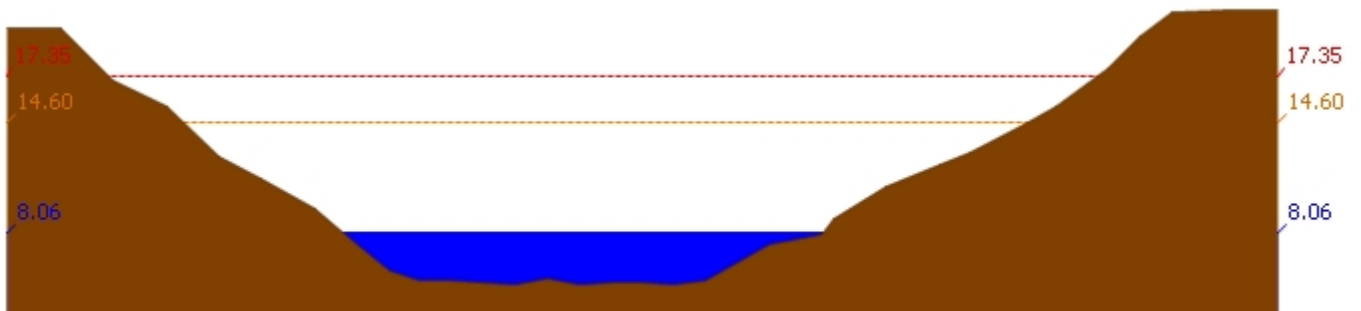
สถานี 120109T แม่น้ำป่าสักที่ อ.แก่งคอย ต.แก่งคอย อ.แก่งคอย จ.สระบุรี ระดับน้ำ 8.06 ม.รทก.
