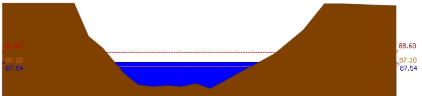
สถานี 120110T แม่น้ำป่าสักที่บ้านวังโบสถ์ ต.วังโบสถ์ อ.หนองไผ่ จ.เพชรบูรณ์ ระดับน้ำ 87.54 ม.รทก.
