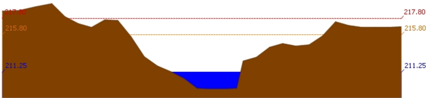
สถานี 120205T แม่น้ำป่าสักที่บ้านอู่กะทาด ต.ศิลา อ.หล่มเก่า จ.เพชรบูรณ์ ระดับน้ำ 211.25 ม.รทก.
