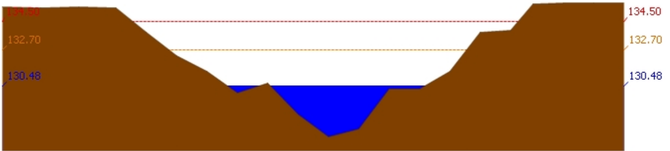
สถานี 120111T แม่น้ำป่าสักที่บ้านจางวาง ต.ลานบัว อ.หล่มสัก จ.เพชรบูรณ์ ระดับน้ำ 130.48 ม.รทก.
