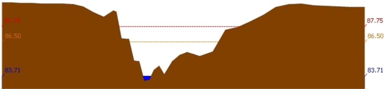
สถานี 110403T หัวขั้วตบเสลาที่บ้านดินแดง ต.ประตู่หิน อ.ลานสัก จ.อุทัยธานี ระดับน้ำ 83.71 ม.รทก.
