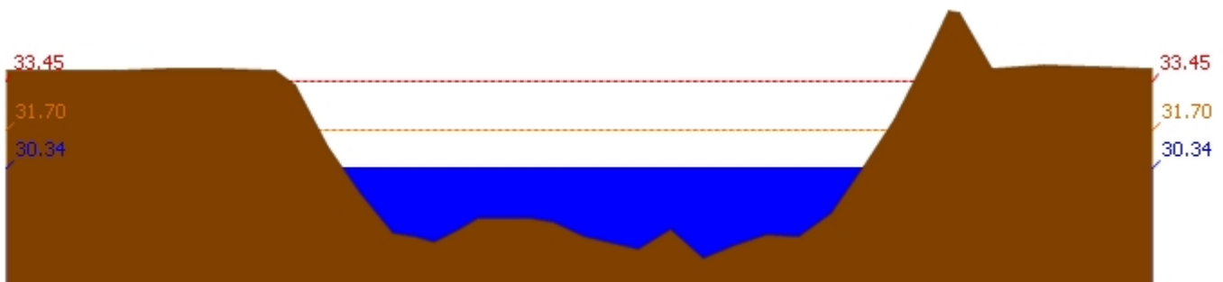
สถานี 110503T แม่น้ำตากแดดที่บ้านหนองขาลาย ต.หนองหลวง อ.สว่างอารมณ์ จ.อุทัยธานี ระดับน้ำ 30.34 ม.รทก.
