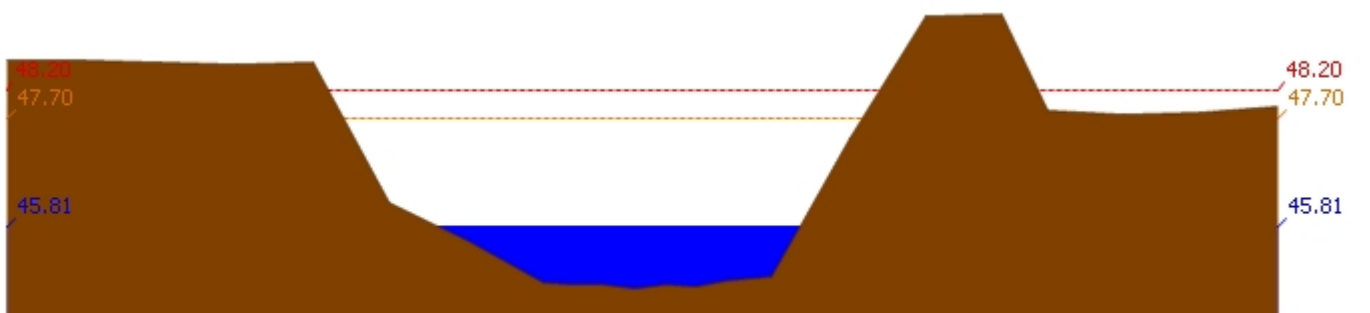
สถานี 110303T คลองโพธิ์ที่บ้านทุ่งสงบ ต.ไม้เขี้ยว อ.สว่างอารมณ์ จ.อุทัยธานี ระดับน้ำ 45.81 ม.รทก.
