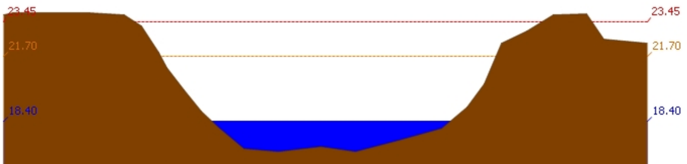
สถานี 110504T แม่น้ำตากแดดที่บ้านบุญลือ ต.เนินแจง อ.เมืองอุทัยธานี จ.อุทัยธานี ระดับน้ำ 18.40 ม.รทก.
