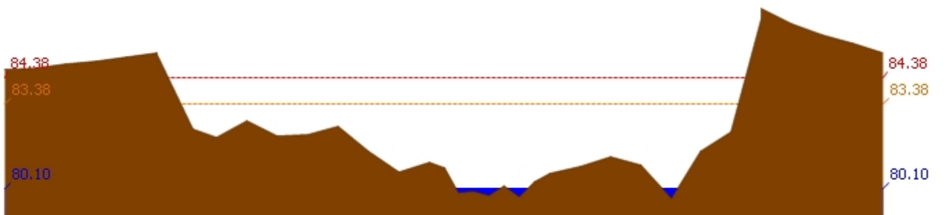
สถานี 062001T คลองสวนหมากที่บ้านน้ำไทรง ต.ท่าขุนราม อ.เมือง จ.กำแพงเพชร ระดับน้ำ 80.10 ม.รทก.
