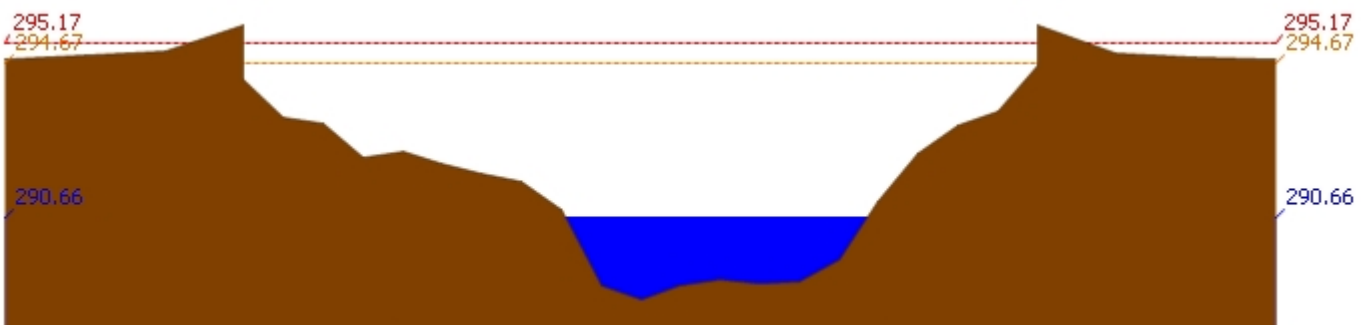
สถานี 060709T น้ำแม่กวางที่ลำพูน ต.เวียงของ อ.เมือง จ.ลำพูน ระดับน้ำ 290.66 ม.รทก.
