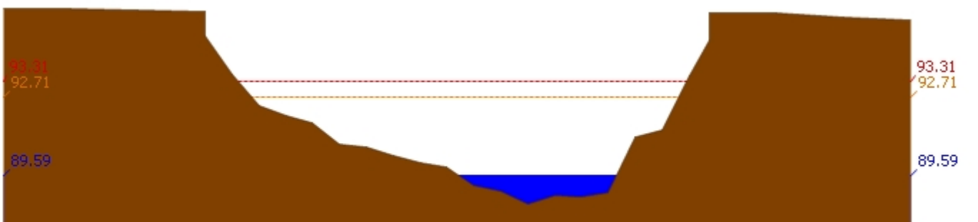
สถานี 061901T คลองแม่ระกาที่บ้านวังชะโอน ต.ท่าไม้ อ.พรานกระต่าย จ.กำแพงเพชร ระดับน้ำ 89.59 ม.รทก.
