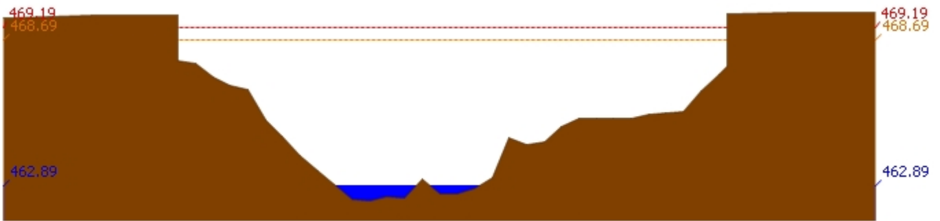
สถานี 060905T น้ำแม่ลี้ที่อำเภอลี้ ต.ลี้ อ.ลี้ จ.ลำพูน ระดับน้ำ 462.89 ม.รทก.
