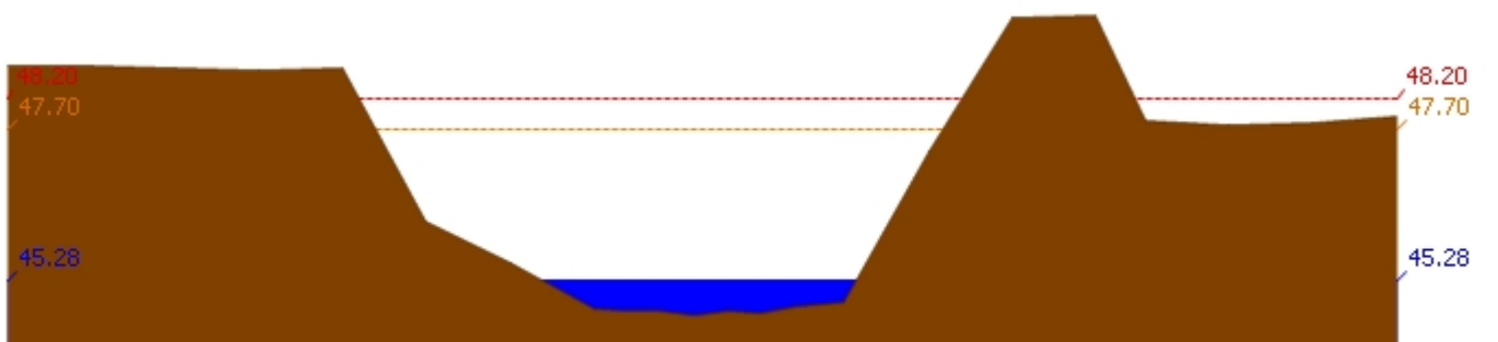
สถานี 110303T คลองโพธิ์ที่บ้านทุ่งสงบ ต.ไม้เขี้ยว อ.สว่างอารมณ์ จ.อุทัยธานี ระดับน้ำ 45.28 ม.รทก.
