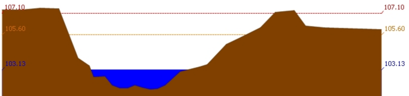
สถานี 110402T ห้วยทับเสลาที่บ้านนาไร่เดียว ต.ลานสัก อ.ลานสัก จ.อุทัยธานี ระดับน้ำ 103.13 ม.รทก.
