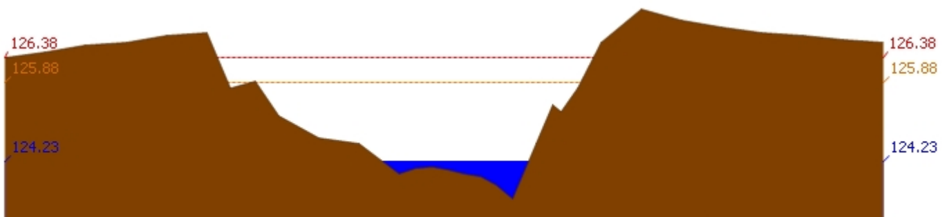
สถานี 110301T คลองโพธิ์ที่บ้านคลองบัวสามัคคี ต.ปางสวรรค์ อ.ชุมตาบง จ.นครสวรรค์ ระดับน้ำ 124.23 ม.รทก.
