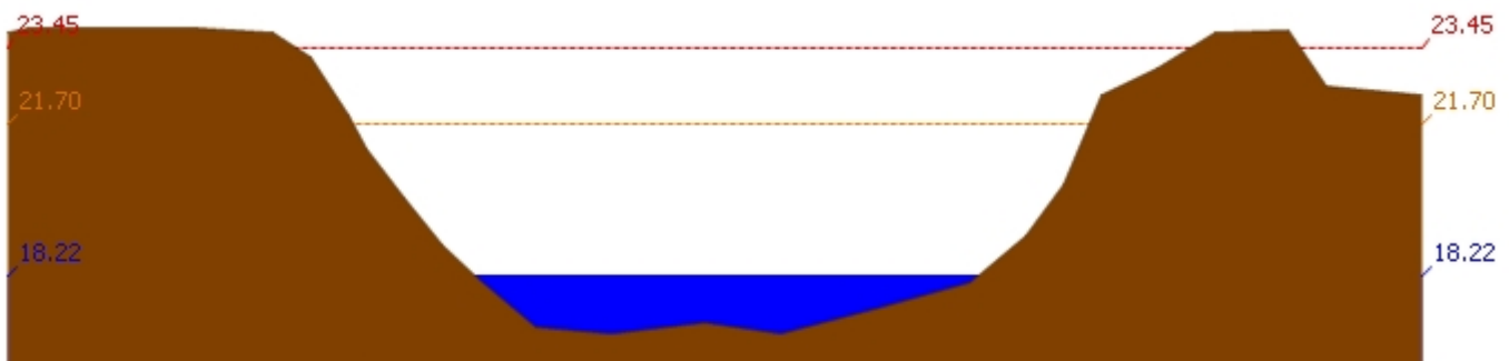
สถานี 110504T แม่น้ำตากแดดที่บ้านบุญลือ ต.เนินแจง อ.เมืองอุทัยธานี จ.อุทัยธานี ระดับน้ำ 18.22 ม.รทก.
