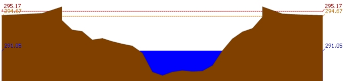
สถานี 060709T น้ำแม่กวางที่ลำพูน ต.เวียงของ อ.เมือง จ.ลำพูน ระดับน้ำ 291.05 ม.รทก.
