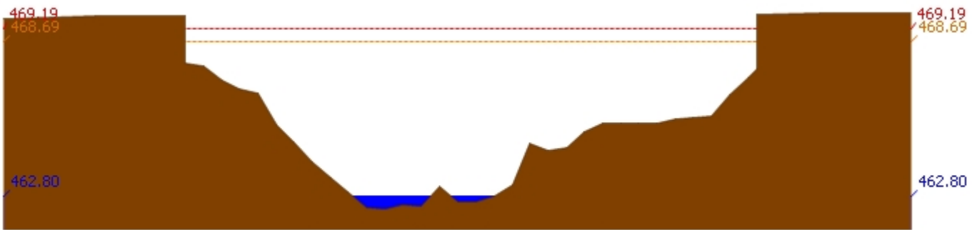
สถานี 060905T น้ำแม่สีที่อำเภอสีคิ้ว อ.สีคิ้ว จ.ลำพูน ระดับน้ำ 462.80 ม.รทก.
