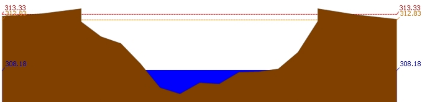
สถานี 060814T น้ำแม่ขานที่บ้านท่าโป่ง ต.บ้านแม อ.สันป่าตอง จ.เชียงใหม่ ระดับน้ำ 308.18 ม.รทก.
