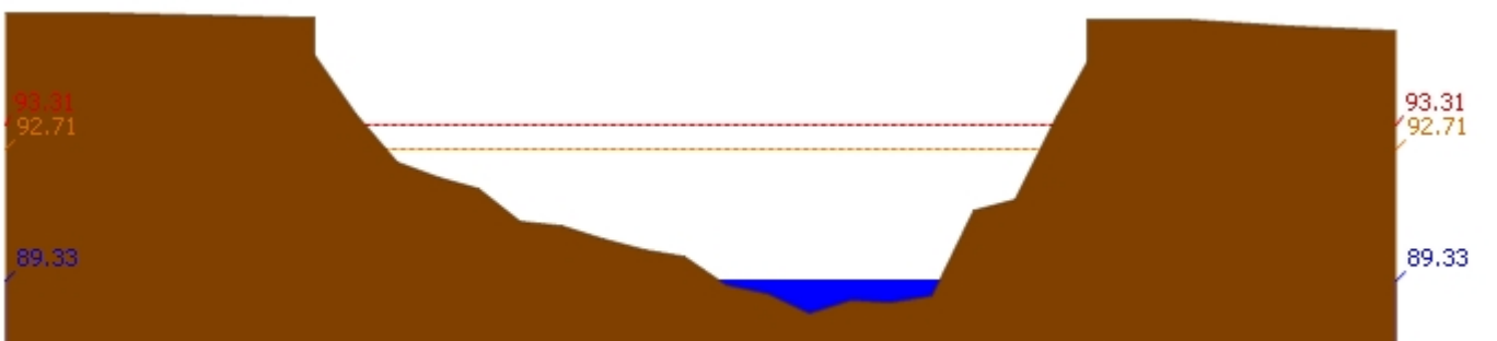
สถานี 061901T คลองแม่ระกาที่บ้านวังชะโอน ต.ท่าไม้ อ.พรานกระต่าย จ.กำแพงเพชร ระดับน้ำ 89.33 ม.รทก.
