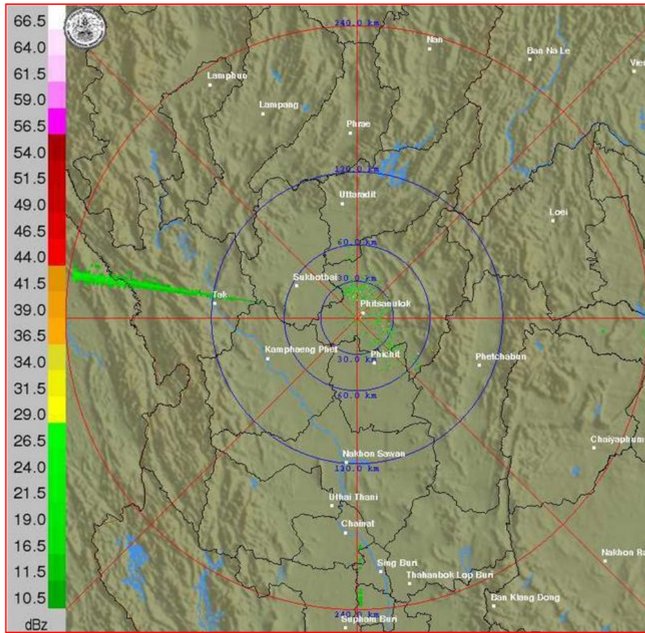
ภาพเรดาร์ตรวจอากาศ “พิษณุโลก” ณ วันที่ 16 พฤษภาคม 2561 (ที่มา : กรมอุตุนิยมวิทยา)
