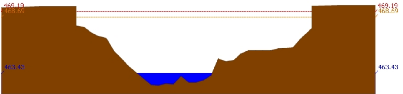
สถานี 060905T น้ำแม่ลี้ที่อำเภอลี้ ต.ลี้ อ.ลี้ จ.ลำพูน ระดับน้ำ 463.43 ม.รทก.
