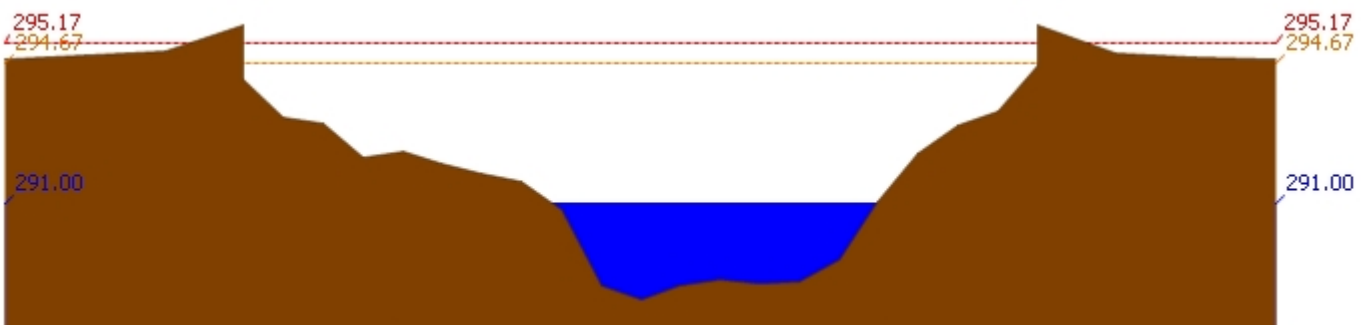
สถานี 060709T น้ำแม่กวงที่ลำพูน ต.เวียงของ อ.เมือง จ.ลำพูน ระดับน้ำ 291.00 ม.รทก.
