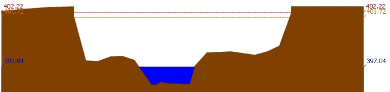
สถานี 060305T น้ำแม่จืดที่บ้านโป่งบัวบาน ต.แม่ปิง อ.พร้าว จ.เชียงใหม่ ระดับน้ำ 397.04 ม.รทก.
