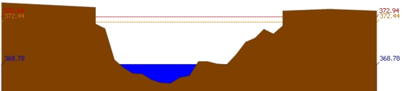
สถานี 060109T แม่น้ำปิงที่บ้านสบอ้อ ต.แม่ระ อ.เชียงดาว จ.เชียงใหม่ ระดับน้ำ 368.78 ม.รทก.
