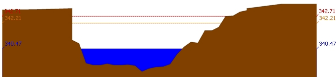
สถานี 070304T น้ำแม่สอยที่บ้านหนองกอก ต.แม่สกก อ.แจ้ห่ม จ.ลำปาง ระดับน้ำ 340.47 ม.รทก.
