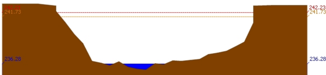
สถานี 070114T แม่น้ำวังที่บ้านปางชัย ต.บ้านเสด็จ อ.เมืองลำปาง จ.ลำปาง ระดับน้ำ 236.28 ม.รทก.
