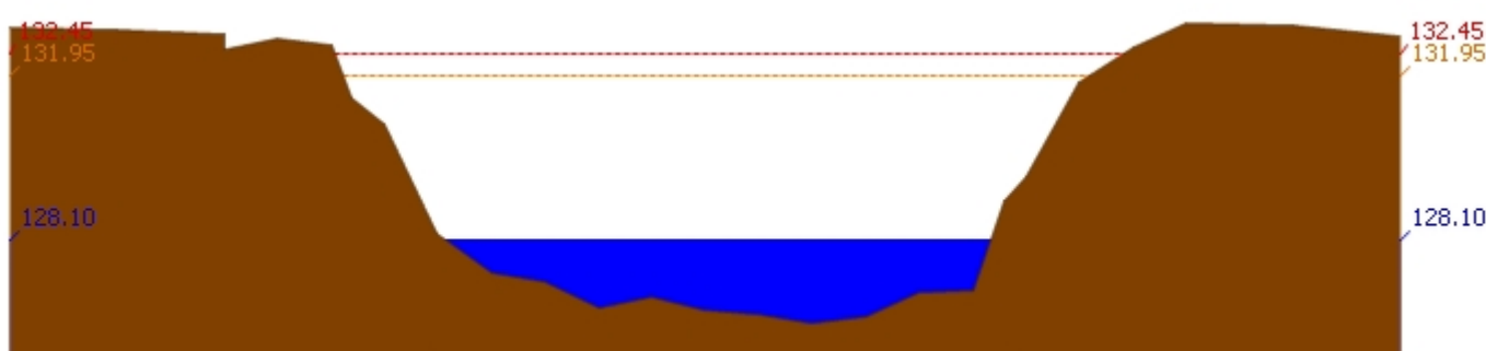
สถานี 070118T แม่น้ำวังที่บ้านแม่สลิด ต.แม่สลิด อ.บ้านตาก จ.ตาก ระดับน้ำ 128.10 ม.รทก.
