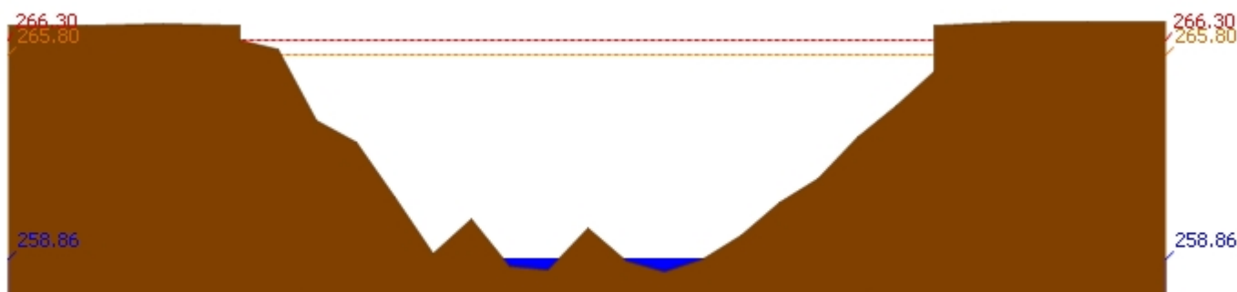
สถานี 070604T น้ำแม่จางที่บ้านสุโหมโขมมงคล ต.หัวเสือ อ.แม่ทะ จ.ลำปาง ระดับน้ำ 258.86 ม.รทก.
