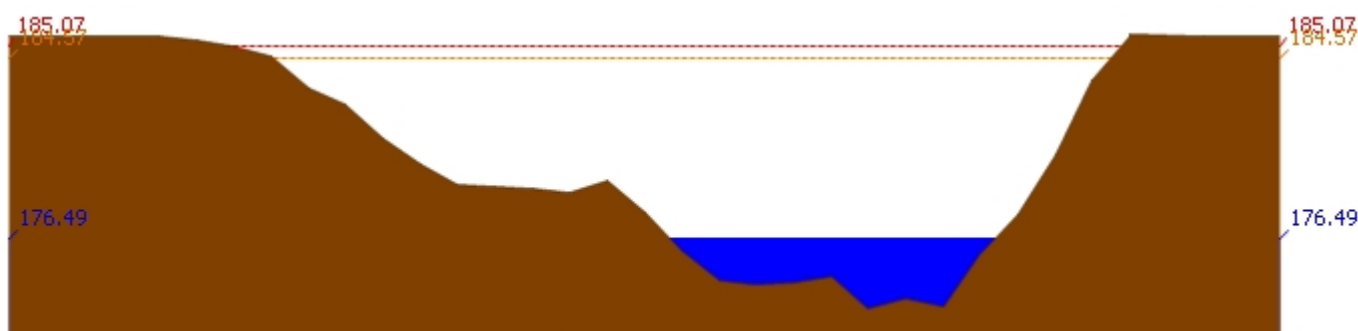
สถานี 070116T แม่น้ำวังที่บ้านแม่เตี๊ยะ ต.แม่ถอด อ.เถิน จ.ลำปาง ระดับน้ำ 176.49 ม.รทก.
