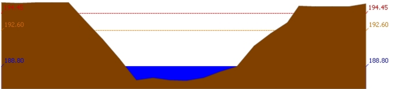
สถานี 120901T ฝายมวกเหล็กที่ อ.มวกเหล็ก ต.มวกเหล็ก อ.มวกเหล็ก จ.สระบุรี ระดับน้ำ 188.80 ม.รทก.
