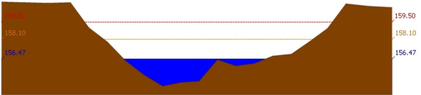
สถานี 120305T ฝายน้ำล้นที่ อ.หล่มเก่า ต.หล่มเก่า อ.หล่มเก่า จ.เพชรบูรณ์ ระดับน้ำ 156.47 ม.รทก.
