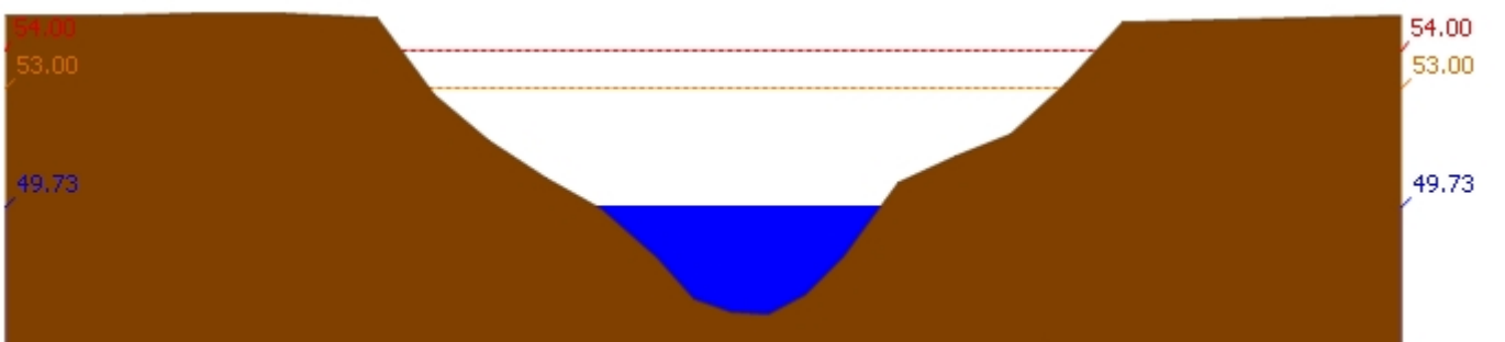
สถานี 120702T ลำสนธิที่บ้านท่าช้าง ต.หนองขาหย่าง อ.ชัยบาดาล จ.ลพบุรี ระดับน้ำ 49.73 ม.รทก.
