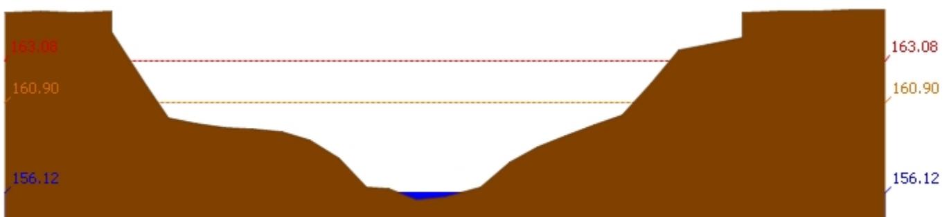
สถานี 120105T แม่น้ำป่าสักที่บ้านวังมลเหนือ ต.ทำอัญญ อ.หล่มสัก จ.เพชรบูรณ์ ระดับน้ำ 156.12 ม.รทก.
