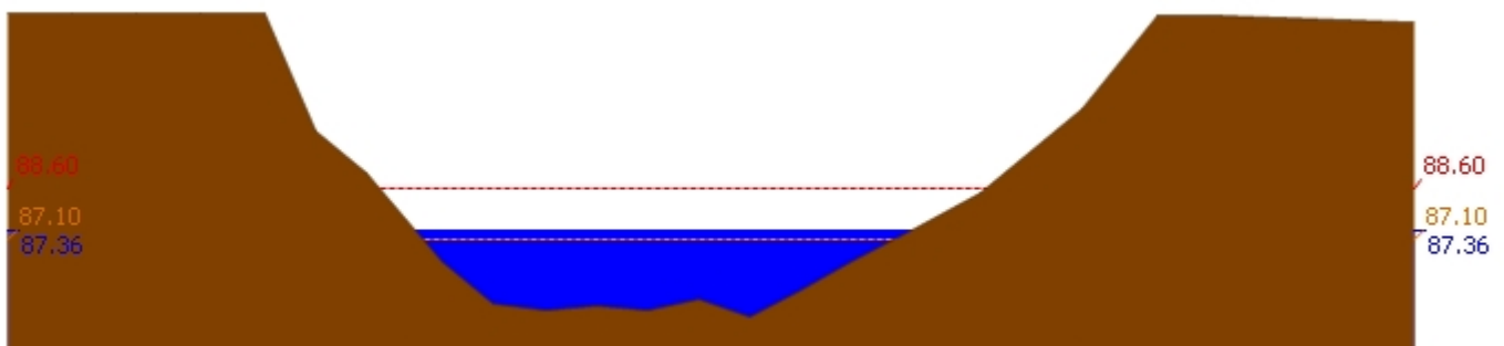
สถานี 120110T แม่น้ำป่าสักที่บ้านวังโบสถ์ ต.วังโบสถ์ อ.หนองไผ่ จ.เพชรบูรณ์ ระดับน้ำ 87.36 ม.รทก.
