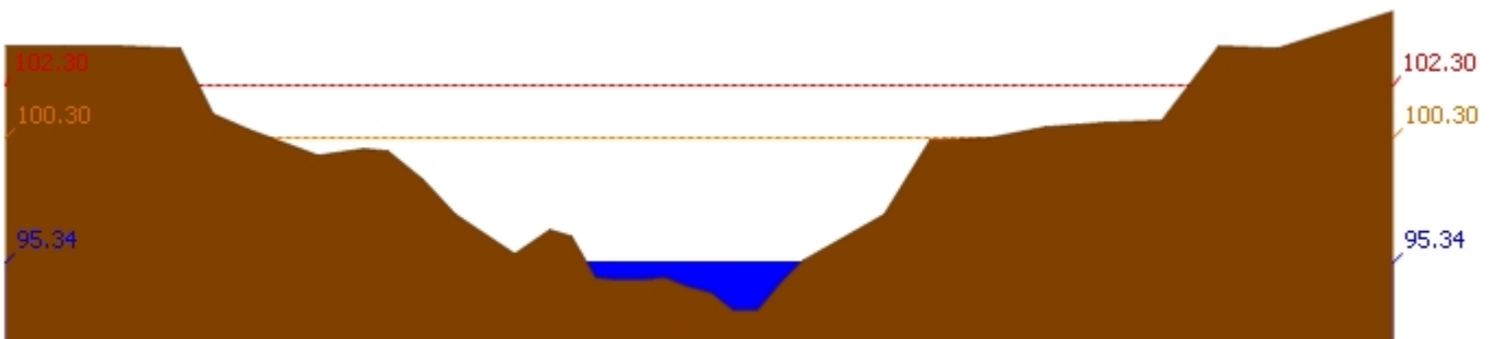
สถานี 120112T แม่น้ำป่าสักที่บ้านหนองแหวน ต.วังมะข่อ อ.เมือง จ.เพชรบูรณ์ ระดับน้ำ 95.34 ม.รทก.
