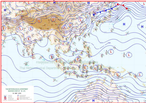
แผนที่อากาศ วันที่ 17 พ.ค. 2561 เวลา 07.00 น.
