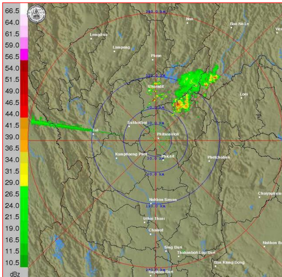
ภาพเรดาร์ตรวจอากาศ “พิชญ์โลก” ณ วันที่ 17 พฤษภาคม 2561 (ที่มา : กรมอุตุนิยมวิทยา)
