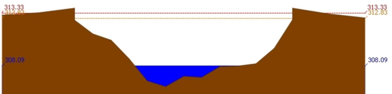
สถานี 060814T น้ำแม่ฆานที่บ้านท่าโป่ง ต.บ้านแม อ.สันป่าตอง จ.เชียงใหม่ ระดับน้ำ 308.09 ม.รทก.
