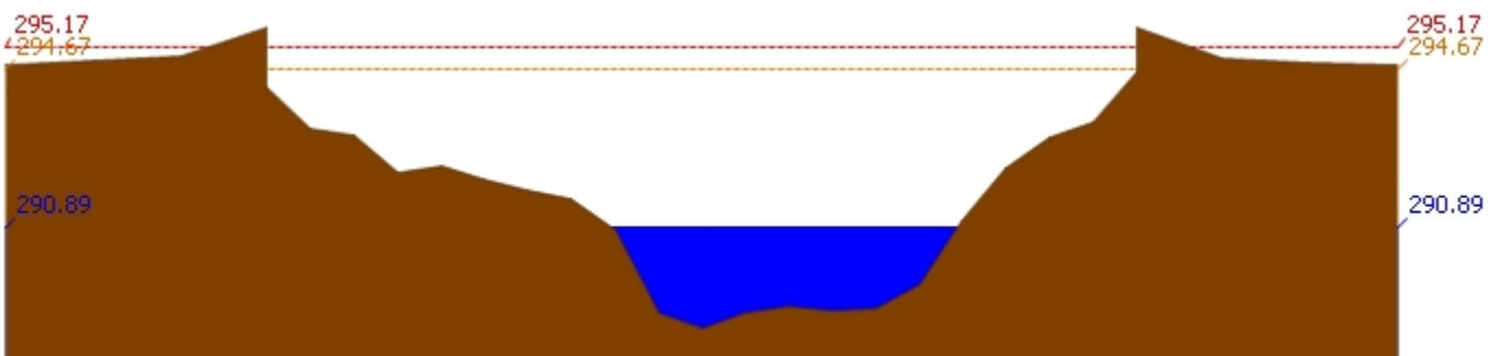
สถานี 060709T น้ำแม่กวงที่ลำพูน ต.เวียงของ อ.เมือง จ.ลำพูน ระดับน้ำ 290.89 ม.รทก.
