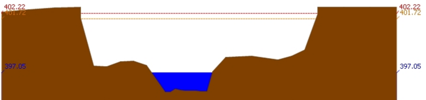
สถานี 060305T น้ำแม่จืดที่บ้านโป่งบัวบาน ต.แม่ปิง อ.พร้าว จ.เชียงใหม่ ระดับน้ำ 397.05 ม.รทก.
