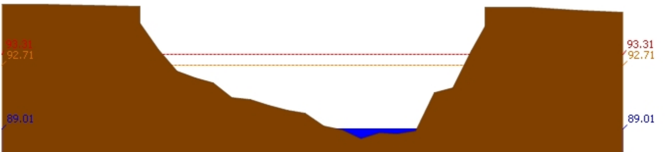
สถานี 061901T คลองแม่ระกาที่บ้านวังชะโอน ต.ท่าไม้ อ.พรานกระต่าย จ.กำแพงเพชร ระดับน้ำ 89.01 ม.รทก.
