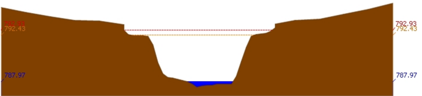
สถานี 061503T น้ำแม่ต้นที่บ้านคอย ต.ยางเปียง อ.อมก๋อย จ.เชียงใหม่ ระดับน้ำ 787.97 ม.รทก.
