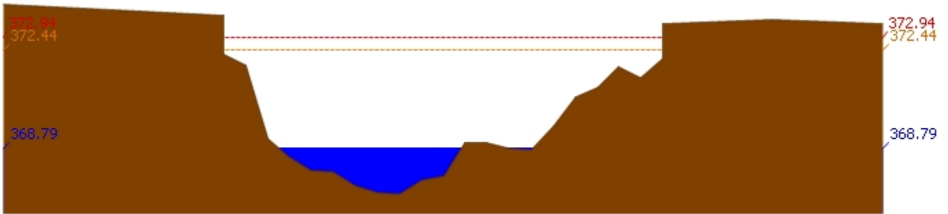
สถานี 060109T แม่ น้ำปิงที่บ้านสบอ้อ ต.แม่่นะ อ.เชียงดาว จ.เชียงใหม่ ระดับน้ำ 368.79 ม.รทก.
