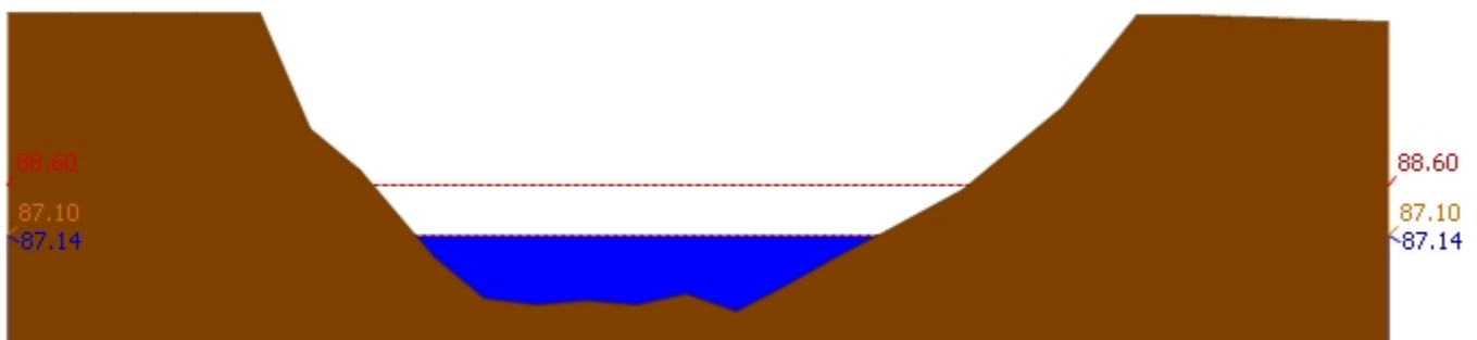
สถานี 120110T แม่น้ำป่าสักที่บ้านวังโบสถ์ ต.วังโบสถ์ อ.หนองไผ่ จ.เพชรบูรณ์ ระดับน้ำ 87.14 ม.รทก.
