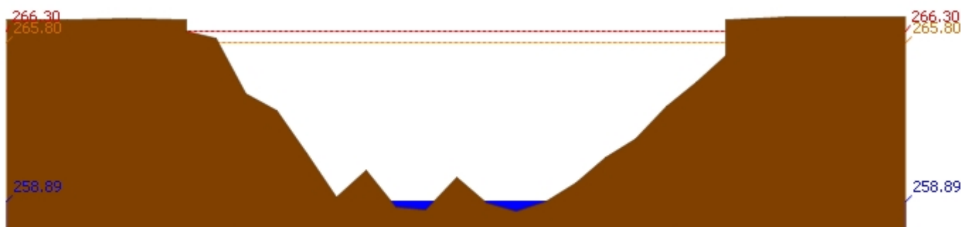
สถานี 070604T น้ำแม่จางที่บ้านสุโหมโขมมงคล ต.หัวเสือ อ.แม่ทะ จ.ลำปาง ระดับน้ำ 258.89 ม.รทก.
