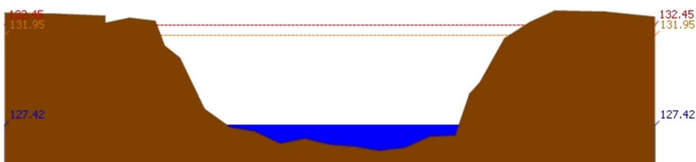
สถานี 070118T แม่น้ำวังที่บ้านแม่สลิด ต.แม่สลิด อ.บ้านตาก จ.ตาก ระดับน้ำ 127.42 ม.รทก.
