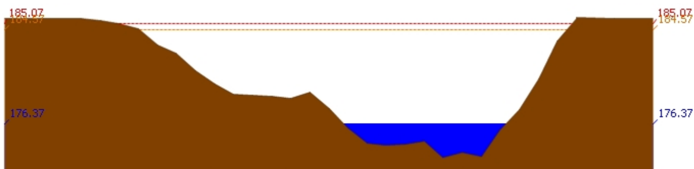
สถานี 070116T แม่น้ำวังที่บ้านแม่เตี๊ยะ ต.แม่ต๋อน อ.เถิน จ.ลำปาง ระดับน้ำ 176.37 ม.รทก.
