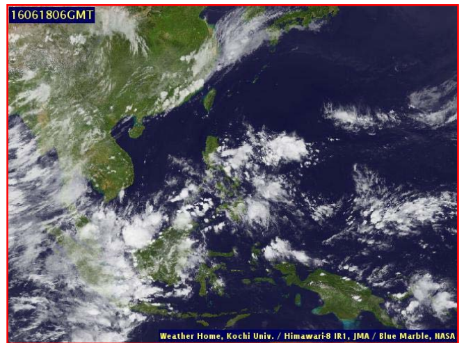
ภาพถ่ายจากดาวเทียม วันที่ ๑๘ มิ.ย. ๒๕๕๙ เวลา ๑๓.๐๐ น.
