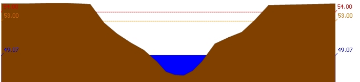
สถานี 120702T ลำสนธิที่บ้านท่าช้าง ต.หนองขาหย่าง อ.ชัยบาดาล จ.ลพบุรี ระดับน้ำ 49.07 ม.รทก.
