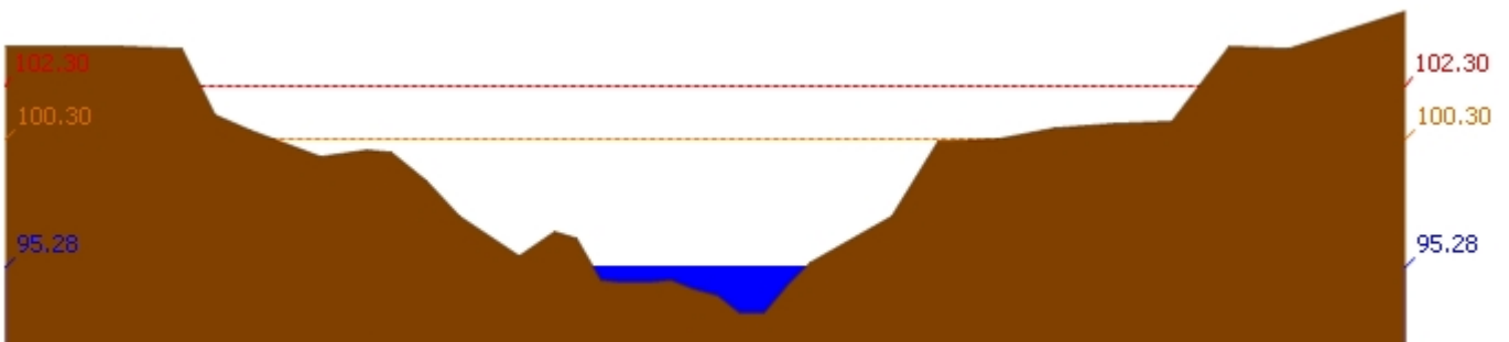
สถานี 120112T แม่น้ำป่าสักที่บ้านหนองแหวน ต.วังมะข่อ อ.เมือง จ.เพชรบูรณ์ ระดับน้ำ 95.28 ม.รทก.
