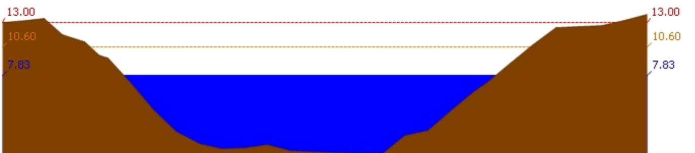
สถานี 120106T แม่น้ำป่าสักที่ อ.เสาไห้ ต.ศาลาวิไทย อ.เสาไห้ จ.สระบุรี ระดับน้ำ 7.83 ม.รทก.
