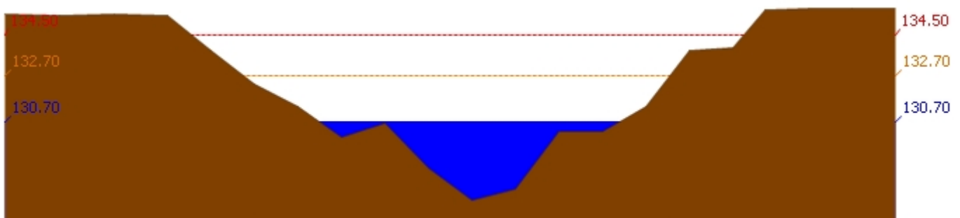
สถานี 120111T แม่น้ำป่าสักที่บ้านจางวาง ต.ลานบ่า อ.หล่มสัก จ.เพชรบูรณ์ ระดับน้ำ 130.70 ม.รทก.
