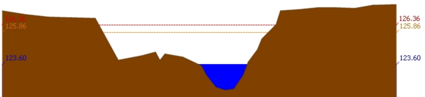
สถานี 110401T ห้วยทับเสลาที่บ้านบึงอ้ายเจียม ต.ระบำ อ.ลานสัก จ.อุทัยธานี ระดับน้ำ 123.60 ม.รทก.
