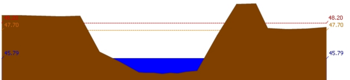
สถานี 110303T คลองโพธิ์ที่บ้านทุ่งสงบ ต.ไม้เขี้ยว อ.สว่างอารมณ์ จ.อุทัยธานี ระดับน้ำ 45.79 ม.รทก.
