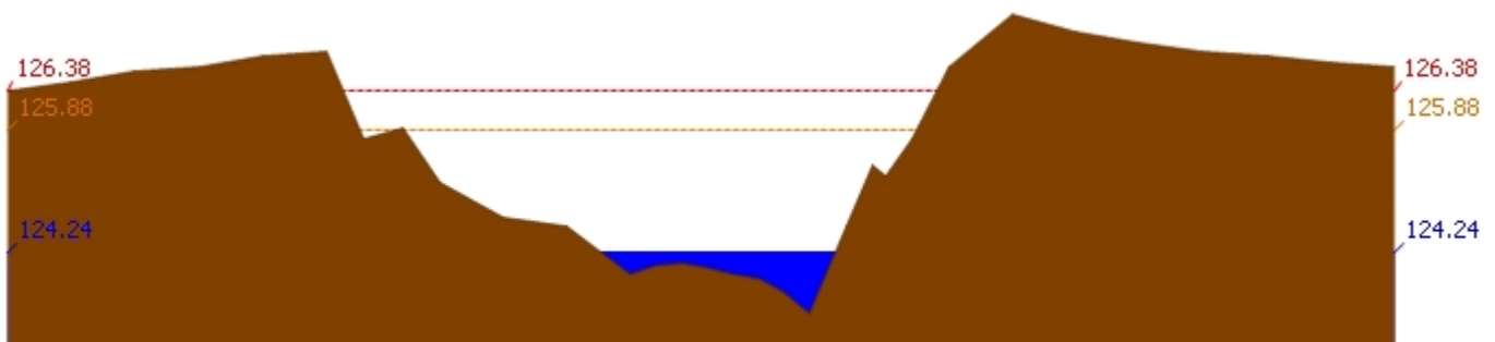
สถานี 110301T คลองโพธิ์ที่บ้านคลองบัวงามสามัคคี ต.ปางสวรรค์ อ.ชุมตาบง จ.นครสวรรค์ ระดับน้ำ 124.24 ม.รทก.
