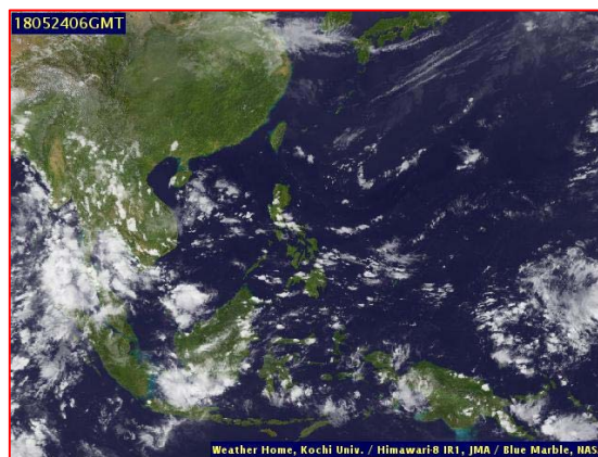
ภาพถ่ายจากดาวเทียม วันที่ ๒๔ พ.ค. ๒๕๖๑ เวลา ๑๓.๐๐ น.
