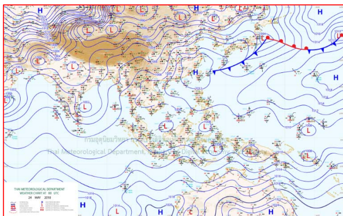
แผนที่อากาศ วันที่ ๒๔ พ.ค. ๒๕๖๑ เวลา ๐๗.๐๐ น.
