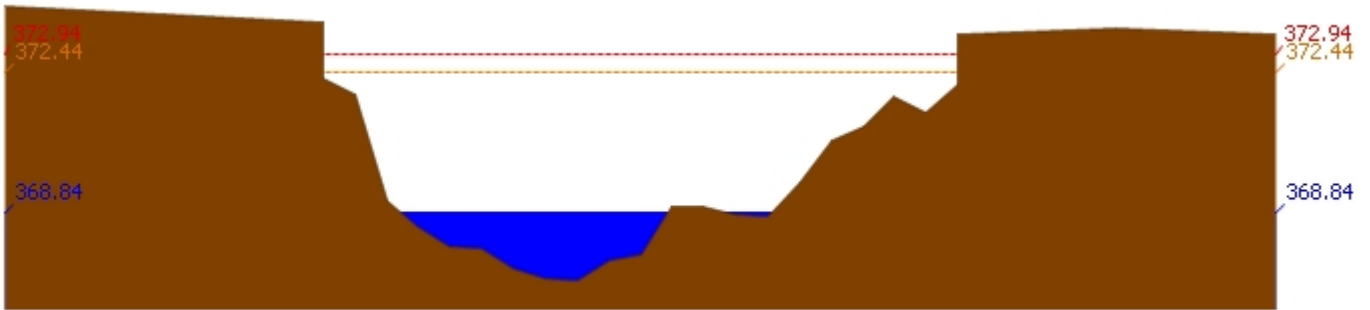
สถานี 060109T แม่ น้ำปิงที่บ้านสบอ้อ ต.แม่ระ อ.เชียงดาว จ.เชียงใหม่ ระดับน้ำ 368.84 ม.รทก.
