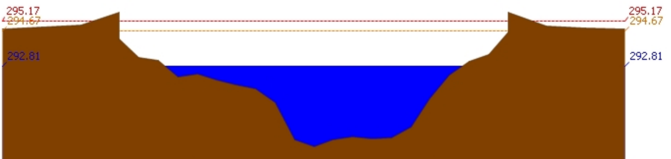
สถานี 060709T น้ำแม่กวงที่ลำพูน ต.เวียงของ อ.เมือง จ.ลำพูน ระดับน้ำ 292.81 ม.รทก.
