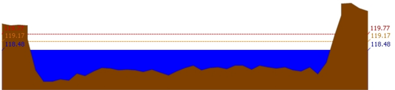
สถานี 060111T แม่น้ำปิงที่บ้านปากร่องห้วยจี่ ต.ตากออก อ.บ้านตาก จ.ตาก ระดับน้ำ 118.48 ม.รทก.
