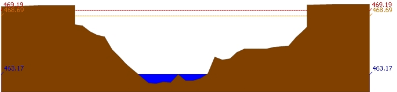
สถานี 060905T น้ำแม่ลี้ที่อำเภอลี้ ต.ลี้ อ.ลี้ จ.ลำพูน ระดับน้ำ 463.17 ม.รทก.
