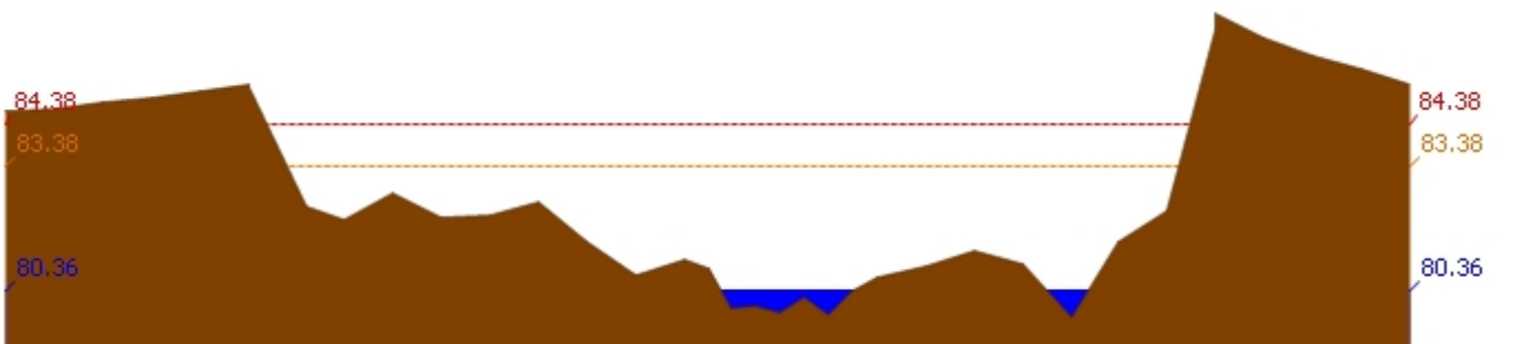
สถานี 062001T คลองสวนหมากที่บ้านน้ำไทรง ต.ท่าขุนราม อ.เมือง จ.กำแพงเพชร ระดับน้ำ 80.36 ม.รทก.
