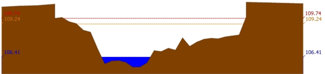
สถานี 061701T ฝายแม่ท้อที่อำเภอเมืองตาก ต.แม่ท้อ อ.เมืองตาก จ.ตาก ระดับน้ำ 106.41 ม.รทก.
