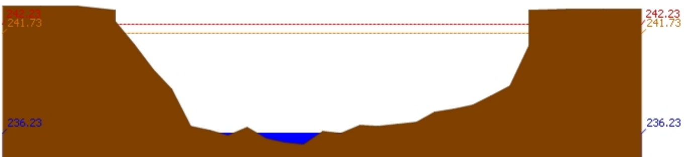
สถานี 070114T แม่น้ำวังที่บ้านปงชัย ต.บ้านเสด็จ อ.เมืองลำปาง จ.ลำปาง ระดับน้ำ 236.23 ม.รทก.
