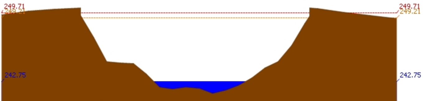
สถานี 070112T แม่น้ำวังที่บ้านบุญนาค ต.บุญนาคพัฒนา อ.เมืองลำปาง จ.ลำปาง ระดับน้ำ 242.75 ม.รทก.
