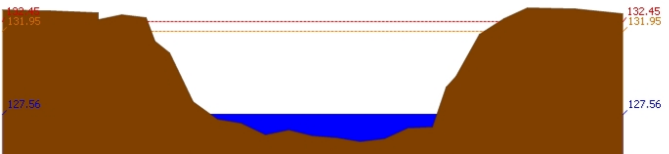
สถานี 070118T แม่น้ำวังที่บ้านแม่สลิด ต.แม่สลิด อ.บ้านตาก จ.ตาก ระดับน้ำ 127.56 ม.รทก.
