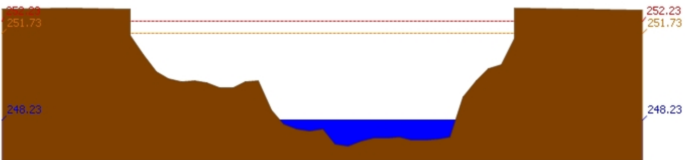
สถานี 070403T น้ำแม่คู่ยที่บ้านแค้ ต.บ้านเป้า อ.เมืองลำปาง จ.ลำปาง ระดับน้ำ 248.23 ม.รทก.
