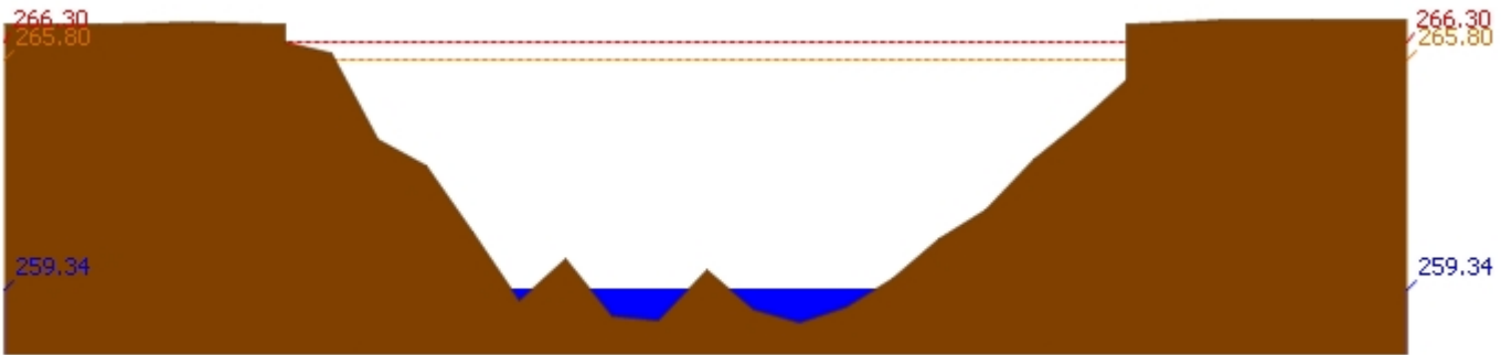
สถานี 070604T น้ำแม่จางที่บ้านสุใหม่โขยมงคล ต.หัวเสือ อ.แม่ทะ จ.ลำปาง ระดับน้ำ 259.34 ม.รทก.
