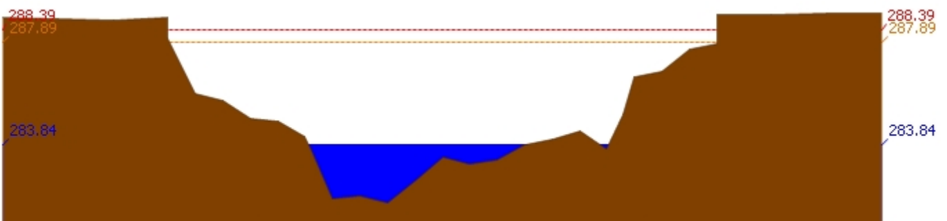
สถานี 070111T แม่บ้านวังที่บ้านแปงโปงชัย ต.บ้านเสา อ.แจ้ห่ม จ.ลำปาง ระดับน้ำ 283.84 ม.รทก.
