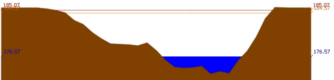
สถานี 070116T แม่น้ำวังที่บ้านแม่เตี๊ยะ ต.แม่ถอด อ.เถิน จ.ลำปาง ระดับน้ำ 176.57 ม.รทก.
