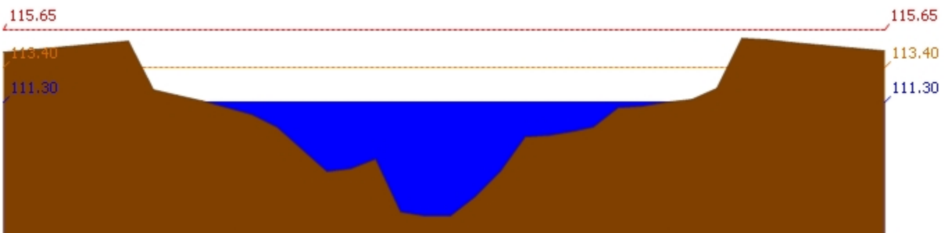
สถานี 120107T แม่น้ำป่าสักที่ อ.เมืองเพชรบูรณ์ ต.นาป่า อ.เมือง จ.เพชรบูรณ์ ระดับน้ำ 111.30 ม.รทก.
