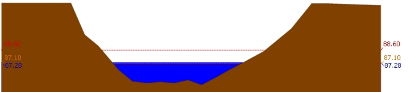
สถานี 120110T แม่น้ำป่าสักที่บ้านวังโบสถ์ ต.วังโบสถ์ อ.หนองไผ่ จ.เพชรบูรณ์ ระดับน้ำ 87.28 ม.รทก.
