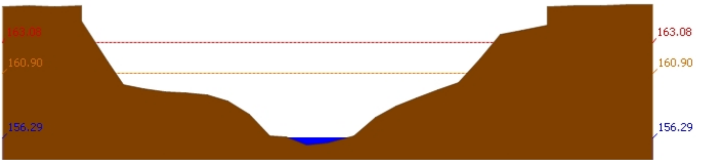
สถานี 120105T แม่น้ำป่าสักที่บ้านวังมเสหนือ ต.ทำอิบุญ อ.หล่มสัก จ.เพชรบูรณ์ ระดับน้ำ 156.29 ม.รทก.
