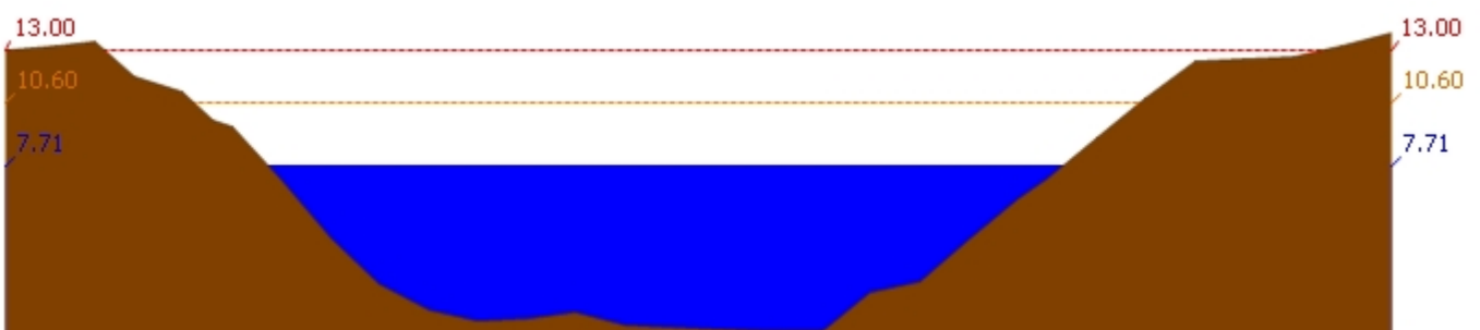
สถานี 120106T แม่น้ำป่าสักที่ อ.เสนาห์ ต.ศาลาวิไทย อ.เสนาห์ จ.สระบุรี ระดับน้ำ 7.71 ม.รทก.
