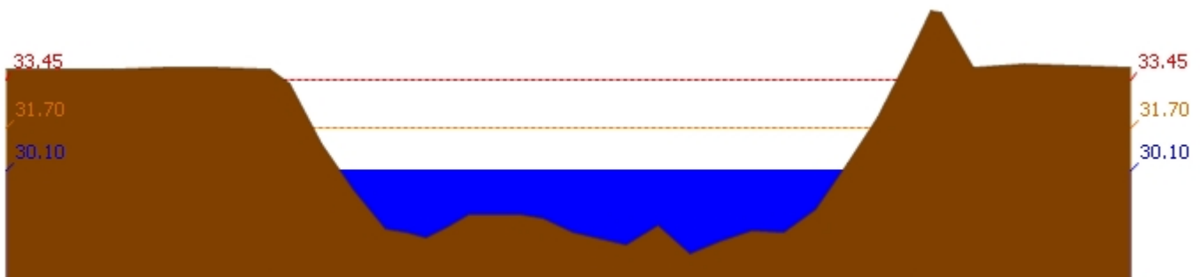
สถานี 110503T แม่น้ำตากแดดที่บ้านหนองขาลาย ต.หนองหลวง อ.สว่างอารมณ์ จ.อุทัยธานี ระดับน้ำ 30.10 ม.รทก.
