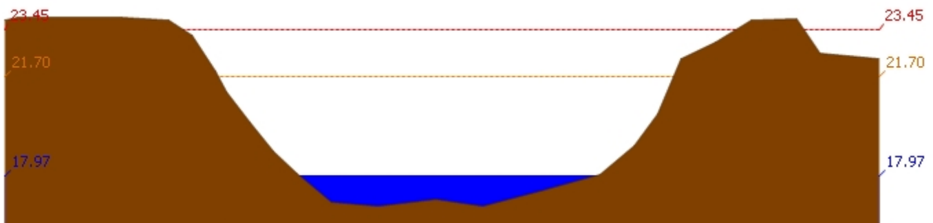
สถานี 110504T แม่น้ำตากแดดที่บ้านบุญลือ ต.เนินแจง อ.เมืองอุทัยธานี จ.อุทัยธานี ระดับน้ำ 17.97 ม.รทก.
