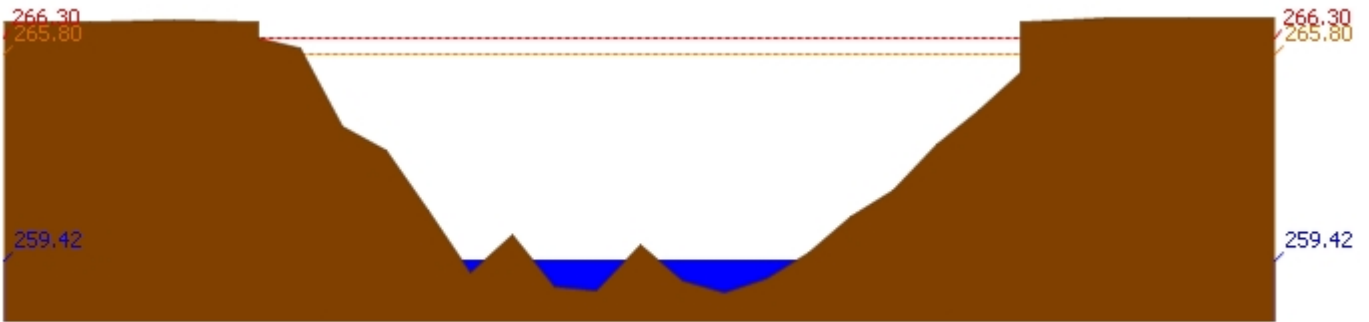
สถานี 070604T น้ำแม่จางที่บ้านสุโหมไชยมงคล ต.หัวเสือ อ.แม่ทะ จ.ลำปาง ระดับน้ำ 259.42 ม.รทก.
