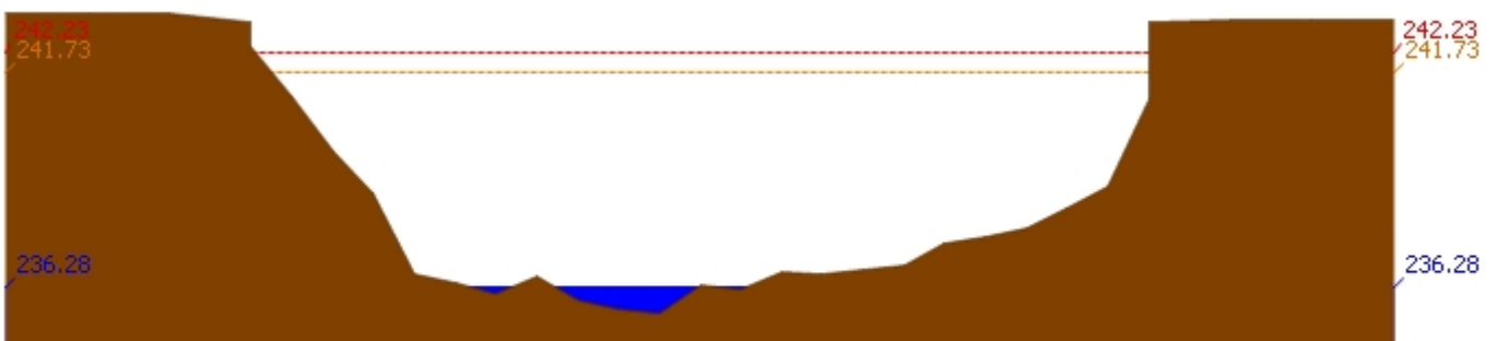
สถานี 070114T แม่น้ำวังที่บ้านปงชัย ต.บ้านเสด็จ อ.เมืองลำปาง จ.ลำปาง ระดับน้ำ 236.28 ม.รทก.
