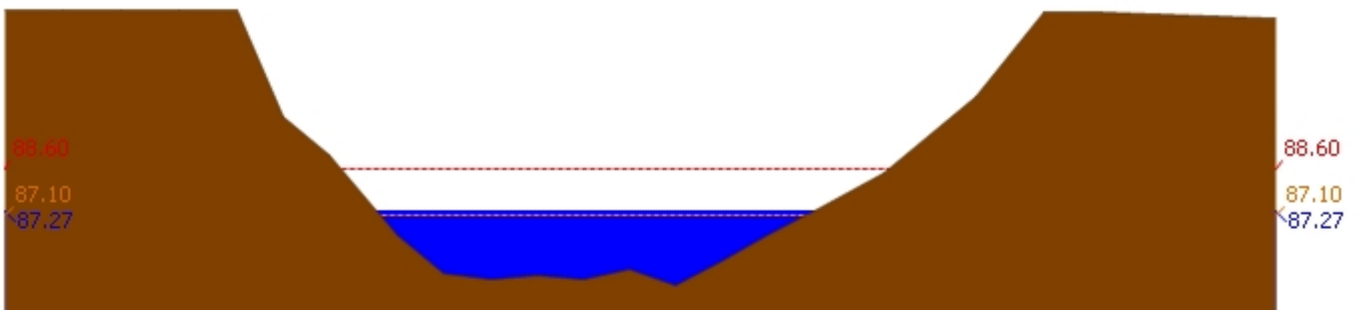
สถานี 120110T แม่น้ำป่าสักที่บ้านวังโบสถ์ ต.วังโบสถ์ อ.หนองไผ่ จ.เพชรบูรณ์ ระดับน้ำ 87.27 ม.รทก.
