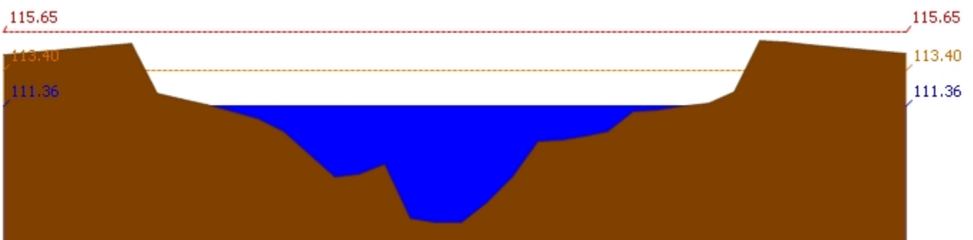
สถานี 120107T แม่น้ำป่าสักที่ อ.เมืองเพชรบูรณ์ ต.นาป่า อ.เมือง จ.เพชรบูรณ์ ระดับน้ำ 111.36 ม.รทก.
