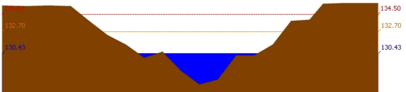
สถานี 120111T แม่น้ำป่าสักที่บ้านจางวาง ต.ลานบัว อ.หล่มสัก จ.เพชรบูรณ์ ระดับน้ำ 130.43 ม.รทก.
