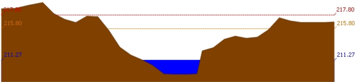
สถานี 120205T แม่น้ำป่าสักที่บ้านอู่กะทาด ต.ศิลา อ.หล่มเก่า จ.เพชรบูรณ์ ระดับน้ำ 211.27 ม.รทก.
