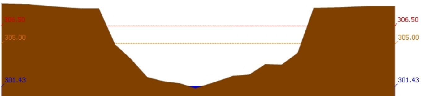
สถานี 120304T หัวน้ำพุที่บ้านกกกะบาก ต.โป่ง อ.ด่านซ้าย จ.เลย ระดับน้ำ 301.43 ม.รทก.
