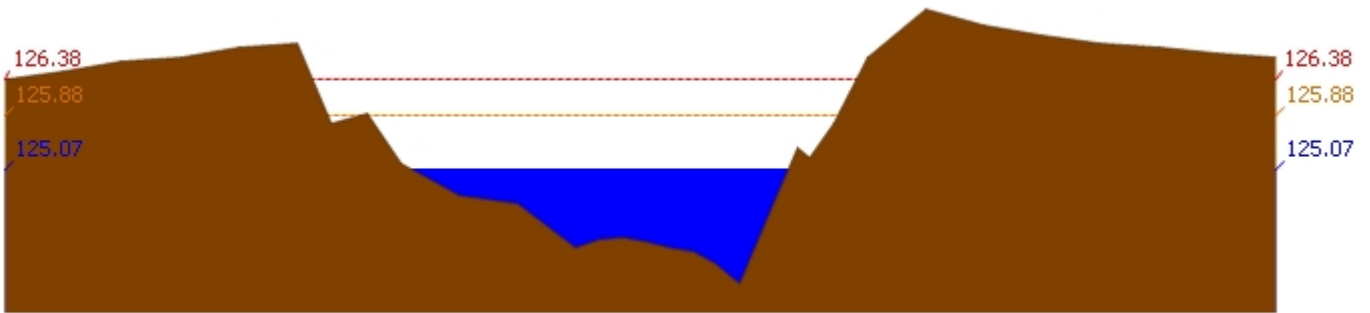
สถานี 110301T คลองโพธิ์ที่บ้านคลองบัวสามัคคี ต.ปางสวรรค์ อ.ชุมตาบง จ.นครสวรรค์ ระดับน้ำ 125.07 ม.รทก.
