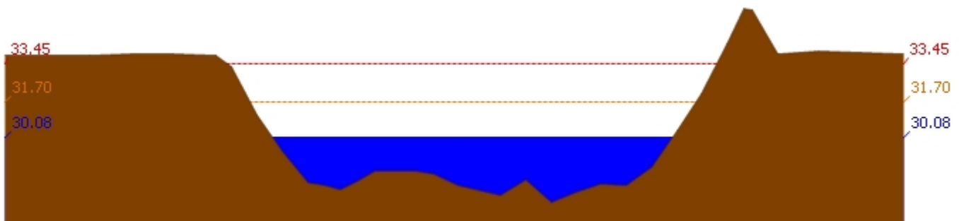
สถานี 110503T แม่น้ำตากแดดที่บ้านหนองขาลาย ต.หนองหลวง อ.สว่างอารมณ์ จ.อุทัยธานี ระดับน้ำ 30.08 ม.รทก.
