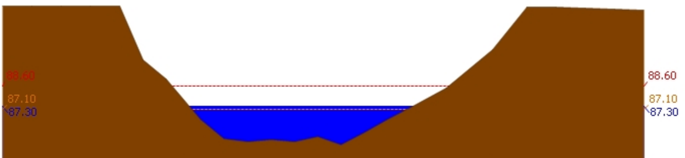
สถานี 120110T แม่น้ำป่าสักที่บ้านวังโบสถ์ ต.วังโบสถ์ อ.หนองไผ่ จ.เพชรบูรณ์ ระดับน้ำ 87.30 ม.รทก.
