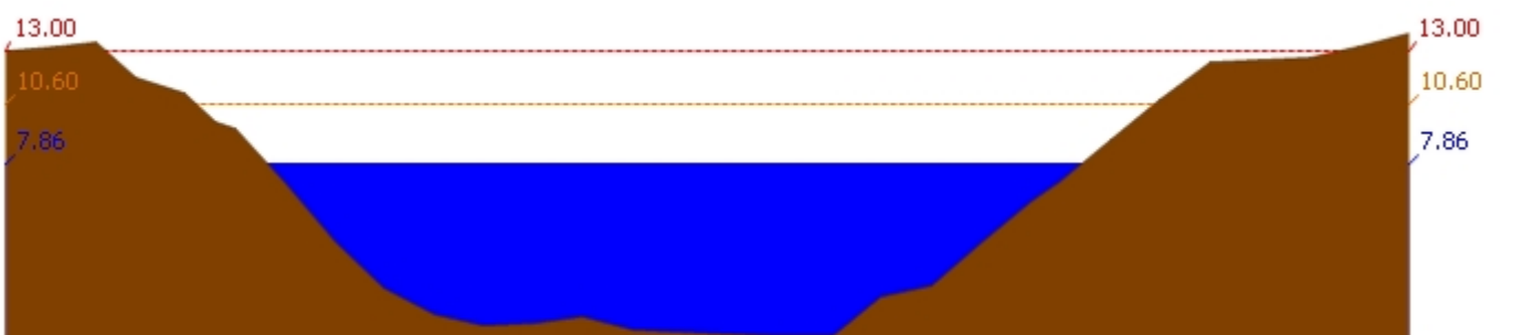
สถานี 120106T แม่น้ำป่าสักที่ อ.เสาไห้ ต.ศาลาวิไทย อ.เสาไห้ จ.สระบุรี ระดับน้ำ 7.86 ม.รทก.
