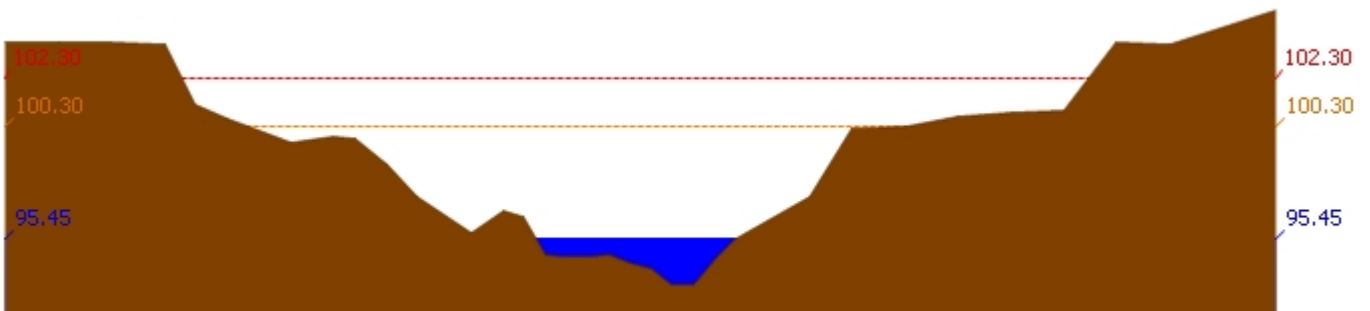
สถานี 120112T แม่น้ำป่าสักที่บ้านหนองแหวน ต.วังมะข่อ อ.เมือง จ.เพชรบูรณ์ ระดับน้ำ 95.45 ม.รทก.
