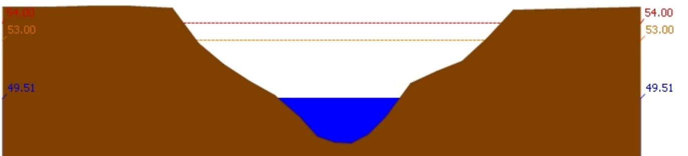
สถานี 120702T ลำสนธิที่บ้านท่าช้าง ต.หนองขายโตะ อ.ชัยบาดาล จ.ลพบุรี ระดับน้ำ 49.51 ม.รทก.
