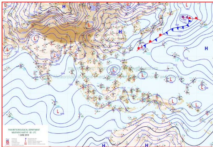
แผนที่อากาศ วันที่ ๑ มิ.ย. ๒๕๖๑ เวลา ๐๗.๐๐ น.
