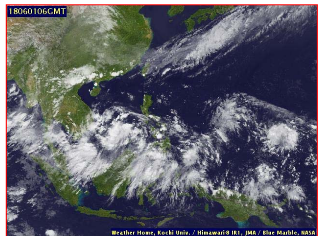
ภาพถ่ายจากดาวเทียม วันที่ ๑ มิ.ย. ๒๕๖๑ เวลา ๑๓.๐๐ น.
