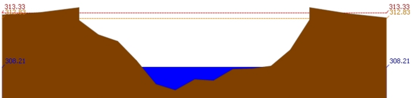
สถานี 060814T น้ำแม่ขานที่บ้านท่าโป่ง ต.บ้านแม อ.สันป่าตอง จ.เชียงใหม่ ระดับน้ำ 308.21 ม.รทก.
