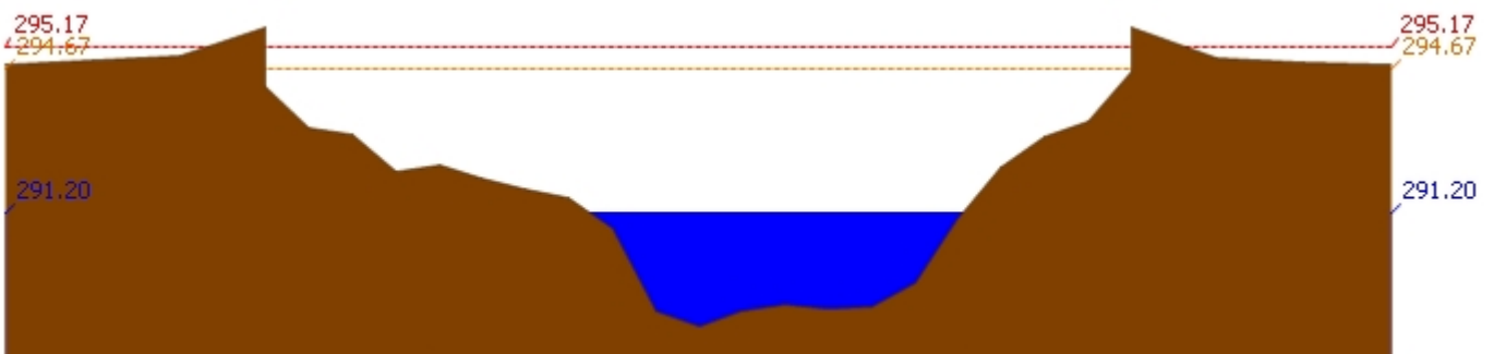
สถานี 060709T น้ำแม่กวางที่ลำพูน ต.เวียงของ อ.เมือง จ.ลำพูน ระดับน้ำ 291.20 ม.รทก.
