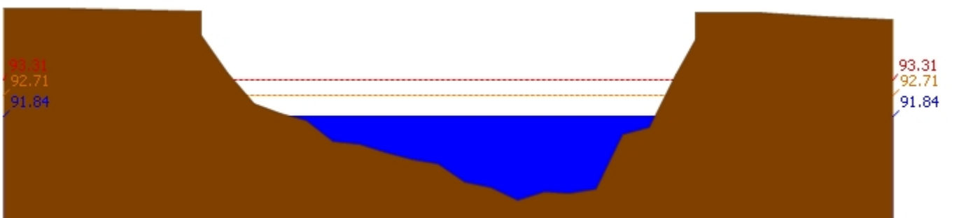
สถานี 061901T คลองแม่ระกาที่บ้านวังชะโอน ต.ท่าไม้ อ.พรานกระต่าย จ.กำแพงเพชร ระดับน้ำ 91.84 ม.รทก.
