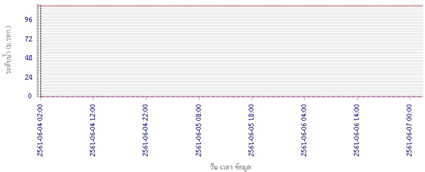
Legend: — ระดับน้ำตรวจวัด (Observed Water Level), - - - ระดับน้ำพยากรณ์ (Forecasted Water Level), - - - ระดับเฝ้าระวัง (Warning Level), - - - ระดับเตือนภัย (Alarm Level)
