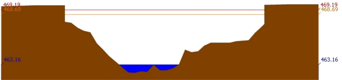
สถานี 060905T น้ำแม่ลี้ที่อำเภอลี้ ต.ลี้ อ.ลี้ จ.ลำพูน ระดับน้ำ 463.16 ม.รทก.
