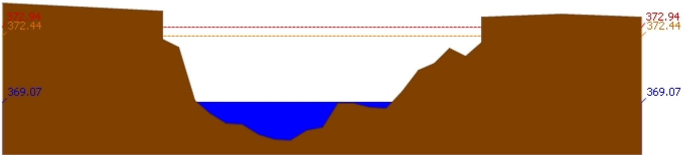
สถานี 060109T แม่น้ำปิงที่บ้านสบอ้อ ต.แม่ระ อ.เชียงดาว จ.เชียงใหม่ ระดับน้ำ 369.07 ม.รทก.
